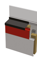
Ouverture / Appui de rive horizontal
