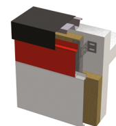
Haut de bardage / finition d'acrotère et couvertine
