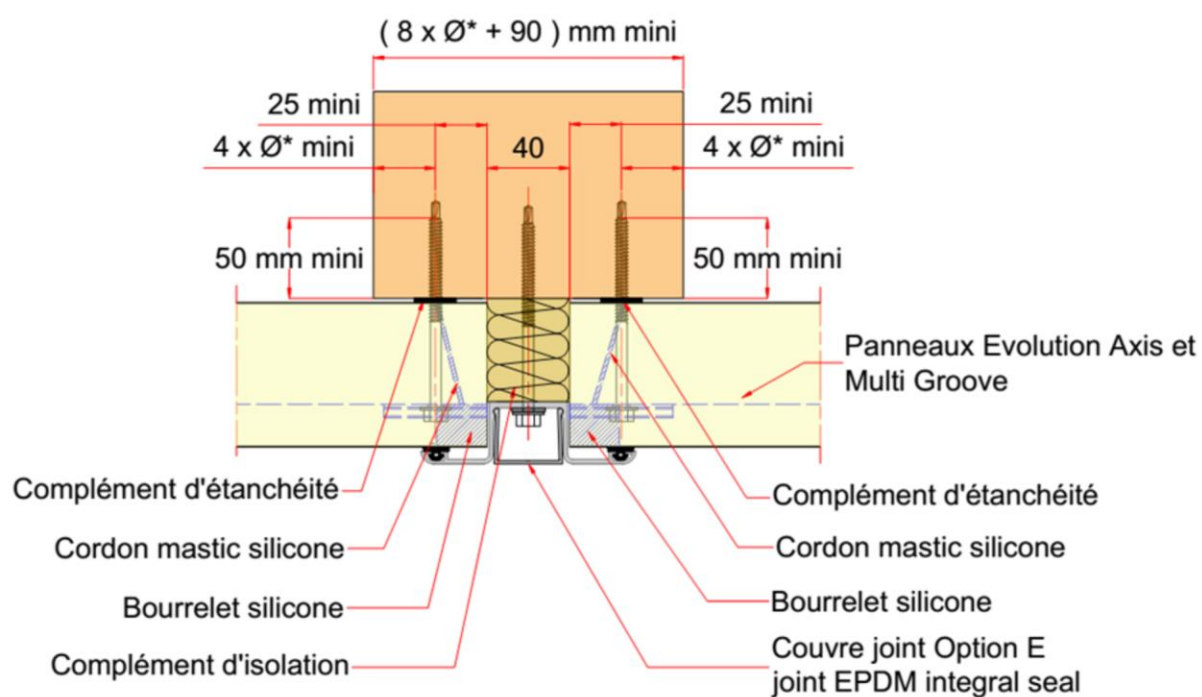
Figure 19 – Exemple d'une jonction verticale en pose horizontale avec panneaux sandwich isolants Evolution Axis ou Multi Groove et couvre-joint option E sur ossature bois
