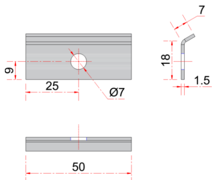
Plaquette de répartition en extrémité de panneau
