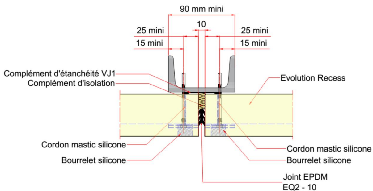
Figure 26 – Exemple d'une jonction verticale en pose horizontale avec panneau sandwich isolant Evolution Recess et joint EPM EQ2-10 sur ossature acier
