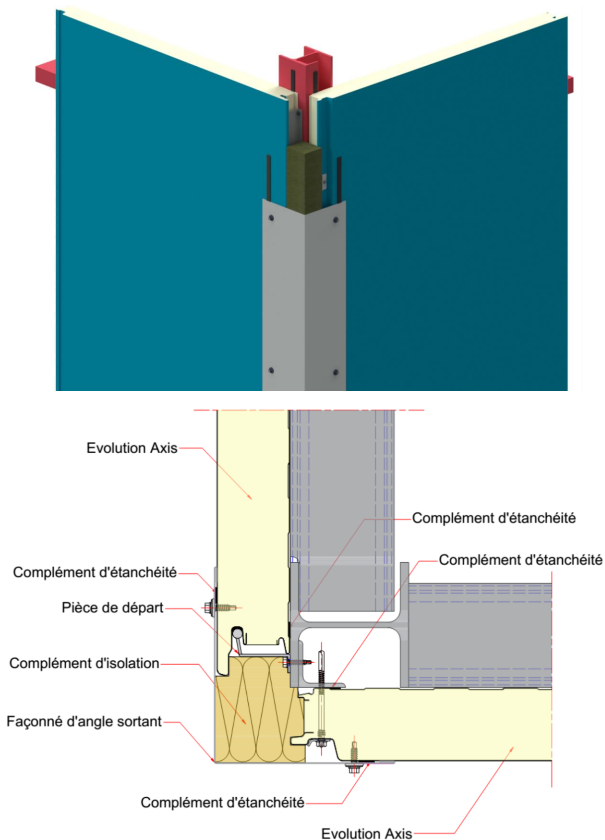
Figure 30 – Exemple d'angle sortant assemblé sur site en pose verticale avec panneau sandwich isolant Evolution Axis
