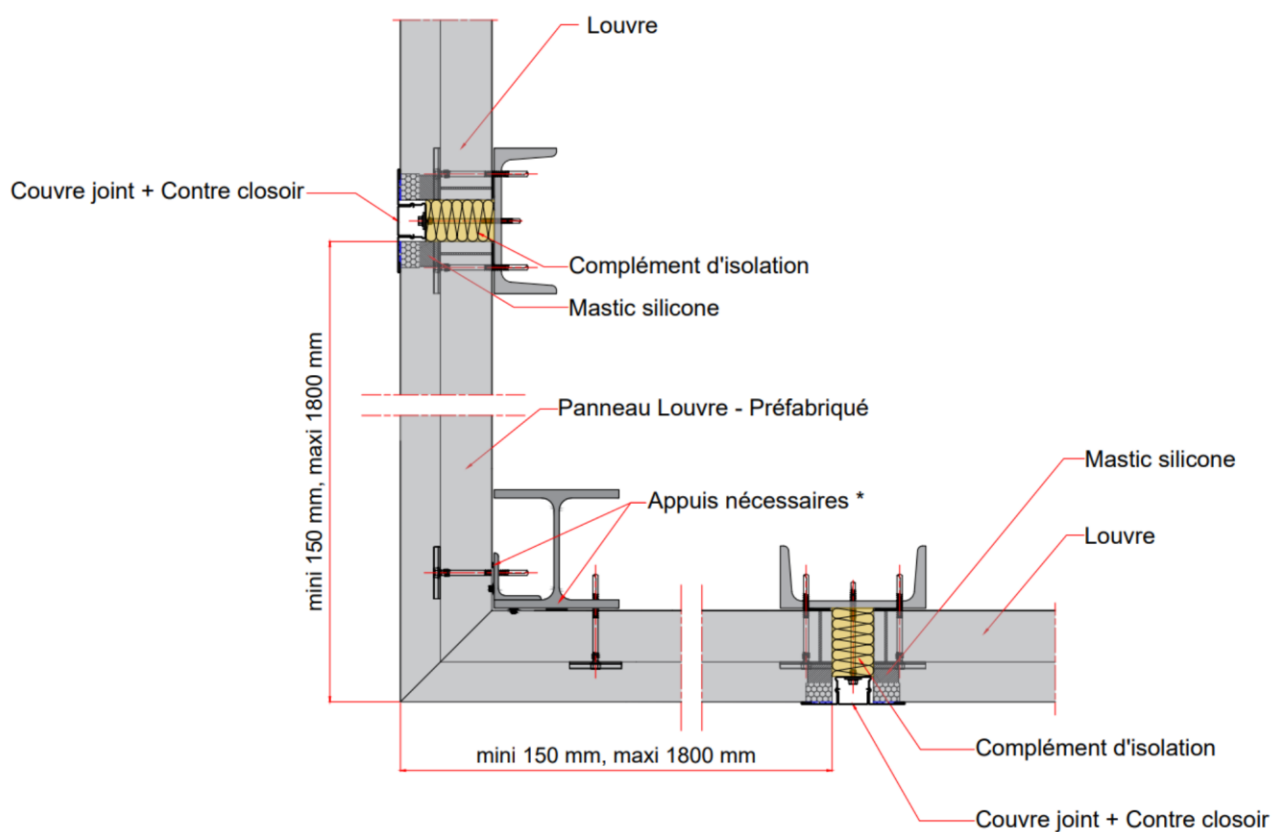
Figure 41 – Exemple d'angle sortant réalisé avec des panneaux préfabriqués Louvre en pose horizontale
