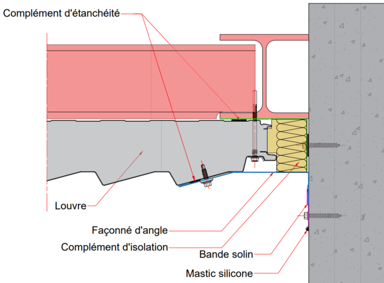
Figure 42 – Exemple d'une rive contre mur avec panneau sandwich isolant louvre en pose verticale
