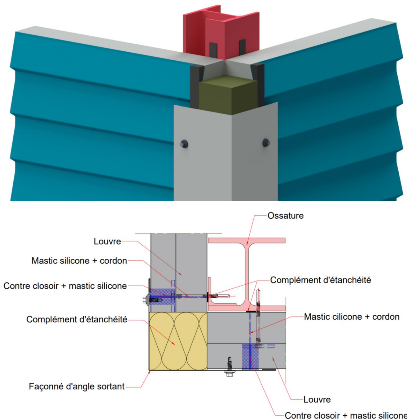
Figure 34 – Exemple d'angle sortant assemblé sur site en pose horizontale avec panneau sandwich isolant Louvre
