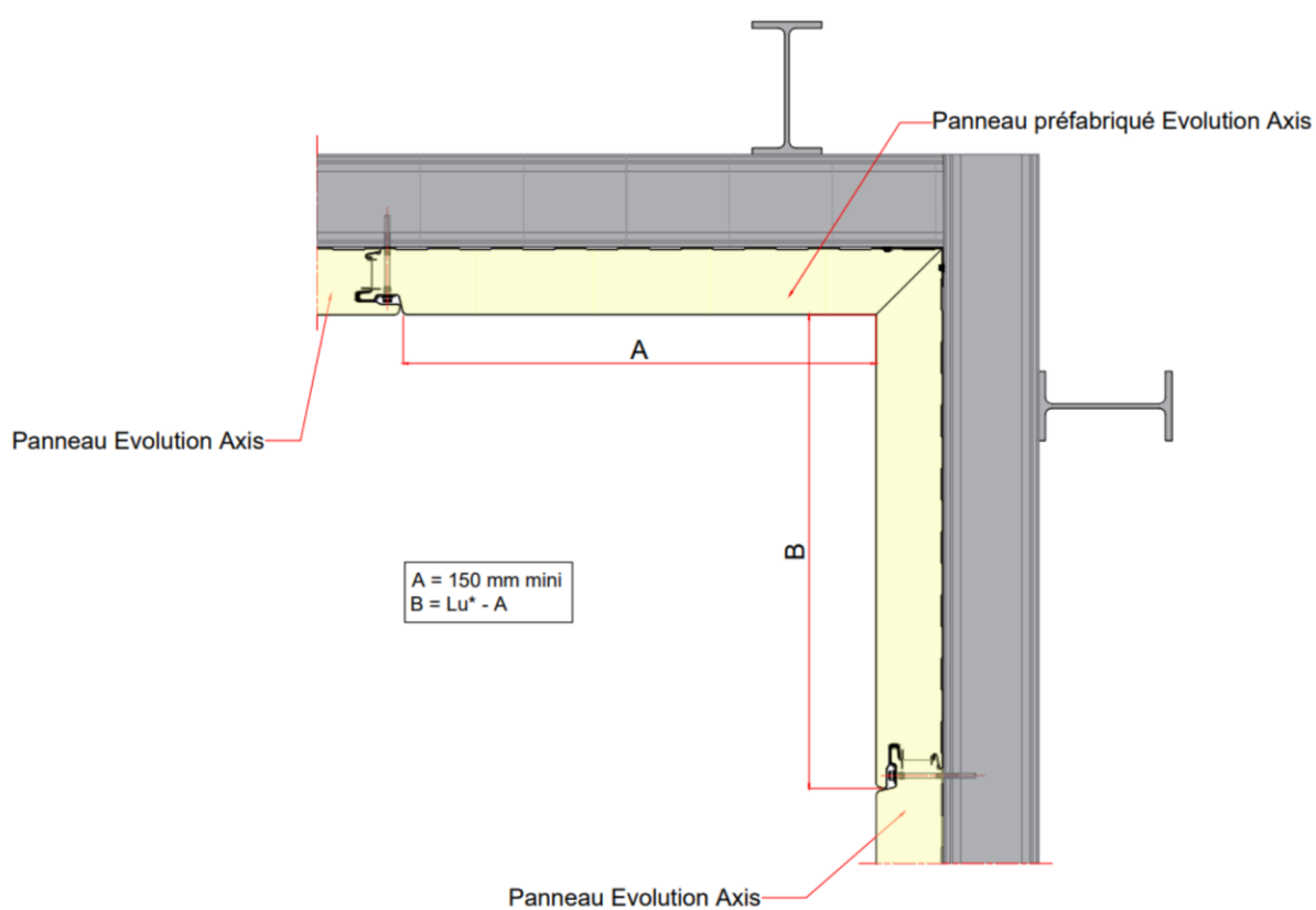
Figure 38 – Exemple d'angle rentrant réalisé avec des panneaux préfabriqués Evolution Axis en pose verticale
