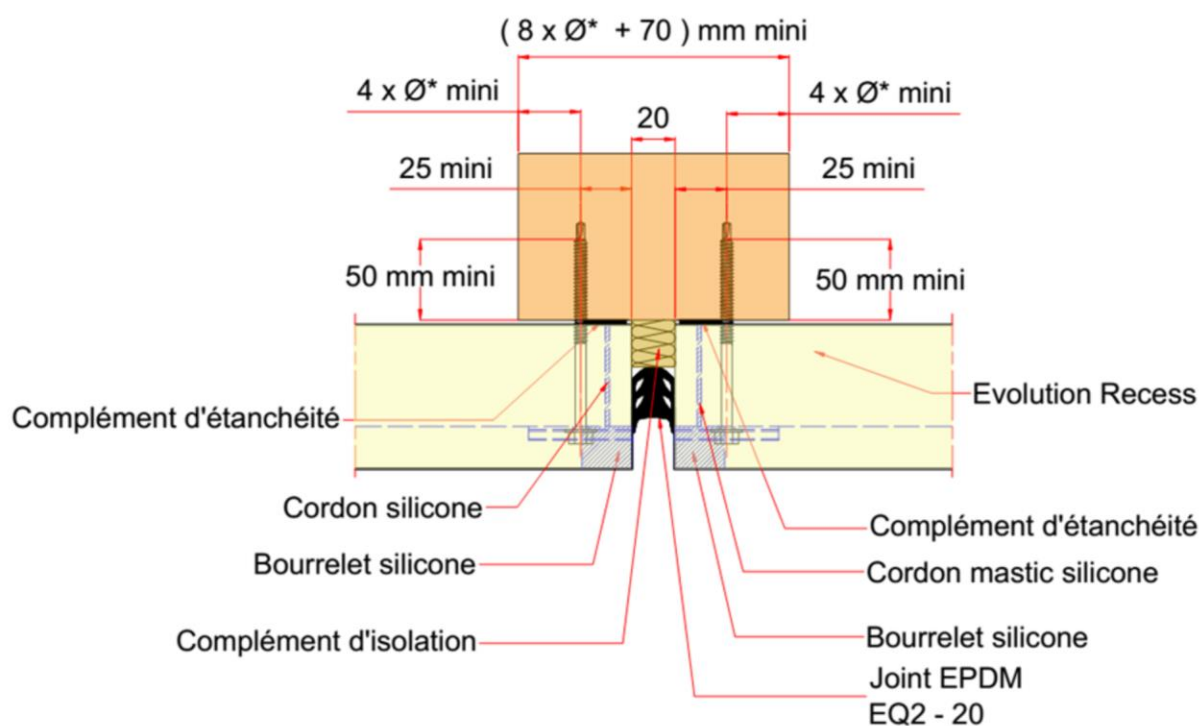
Figure 27 – Exemple d'une jonction verticale en pose horizontale avec panneau sandwich isolant Evolution Recess et joint EPM EQ2-20 sur ossature bois
