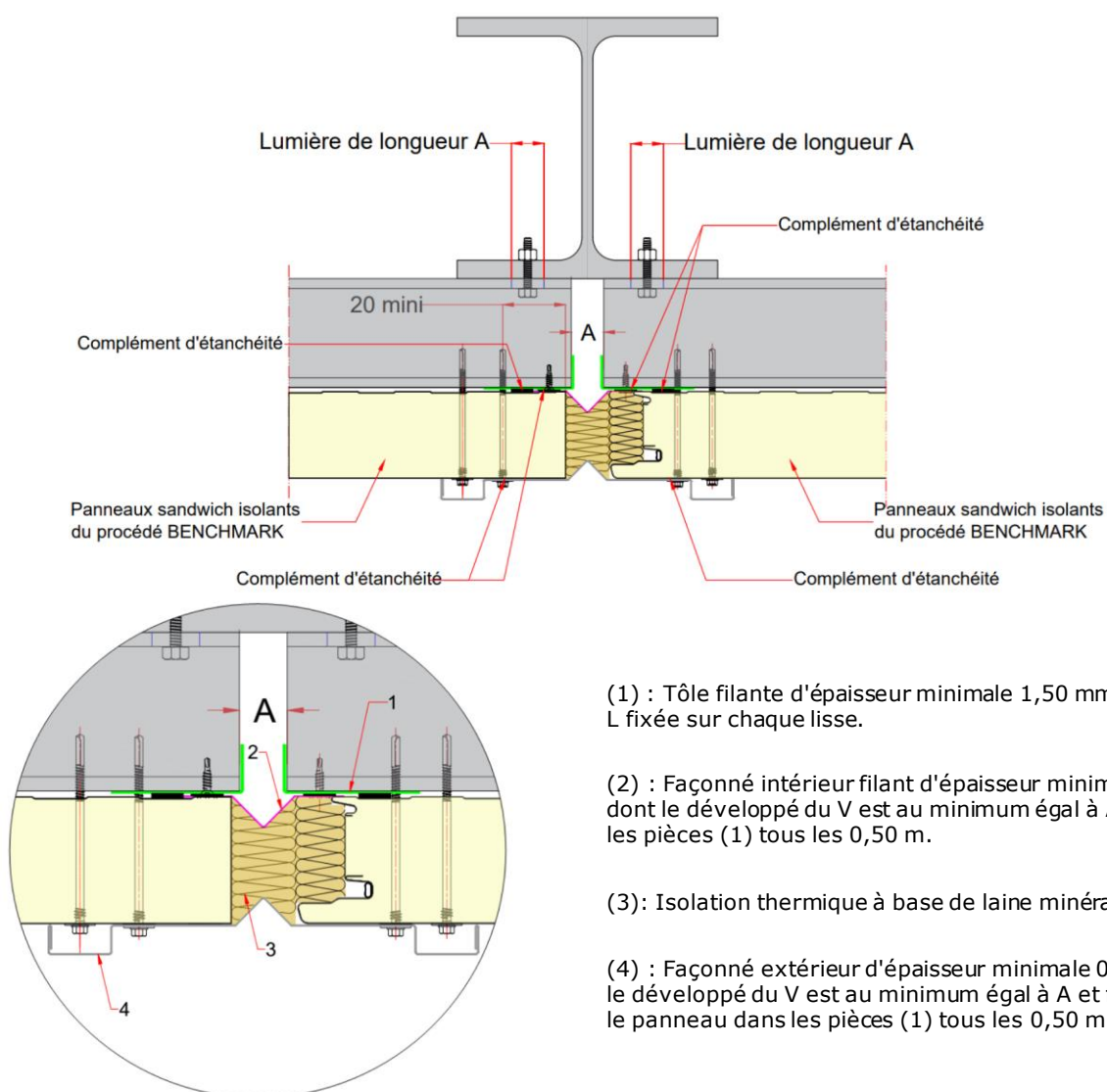
Figure 49 – Exemple d'un joint de dilatation thermique dont le déplacement maximal est de 50 mm avec panneaux sandwich isolants Evolution Axis ou Evolution Multi Groove en pose verticale
