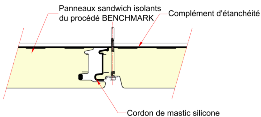
Figure 8 – Dispositions en extrémité haute et basse des panneaux sandwich isolants en pose verticale
