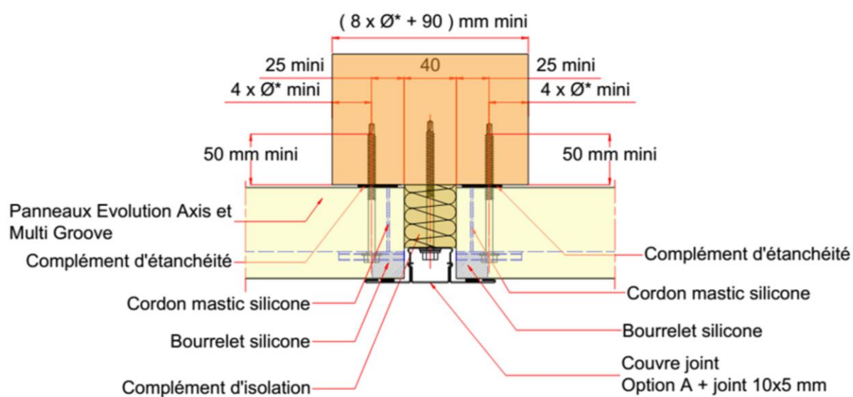
Figure 20 – Exemple d'une jonction verticale en pose horizontale avec panneaux sandwich isolants Evolution Axis ou Multi Groove et couvre-joint option A (Affleurant) sur ossature bois
