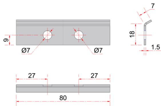
Plaquette de répartition en partie courante de panneau
