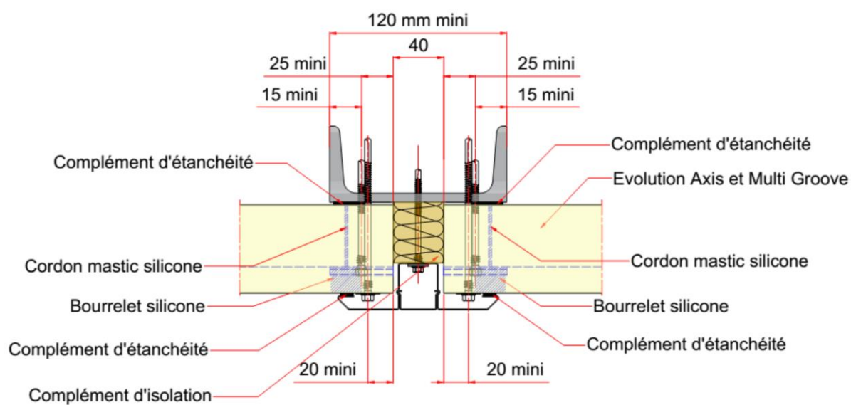
Figure 28 – Exemple d'une jonction verticale en pose horizontale avec panneaux sandwich isolants BENCHMARK et 2 fixations traversantes complémentaires par largeur de panneau – Conception 1 avec panneaux Evolution Axis représenté
