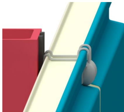
Exemple avec joints mousse 20 x 5 mm disposés sur appuis
