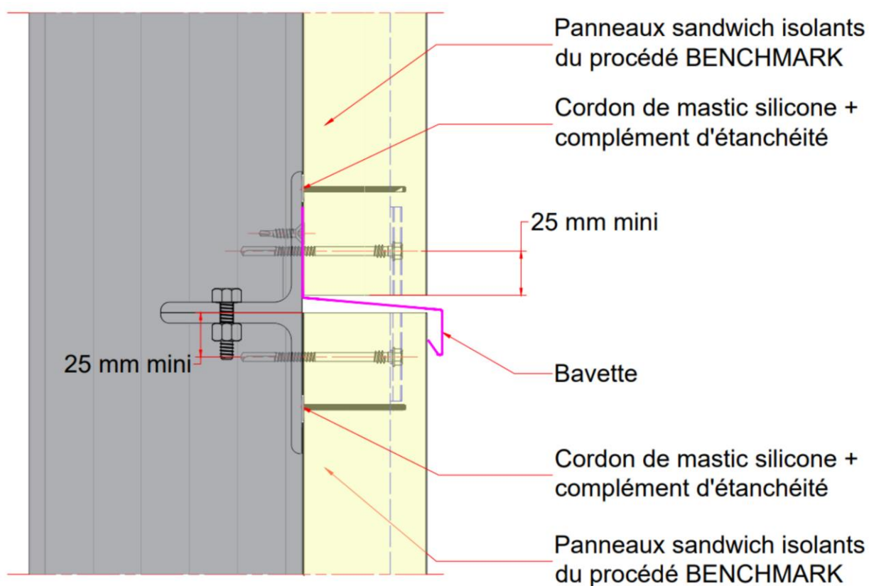
Figure 18 – Jonction horizontale en pose verticale
