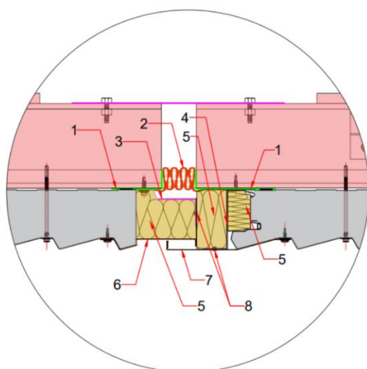
Figure 50 bis – Exemple d'un joint de dilatation dont le déplacement maximal est de 150 mm avec panneau sandwich isolant Louvre en pose verticale
