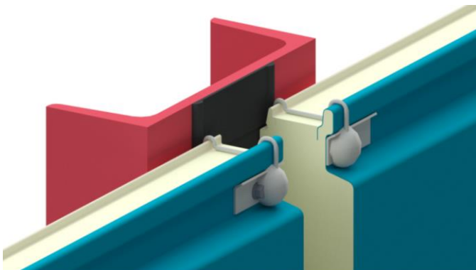
Exemple avec joint EPDM VJ1 ou VJ2 disposé sur appuis
