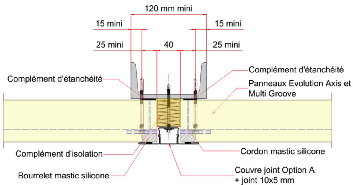
Figure 24 – Exemple d'une jonction verticale en pose horizontale avec panneaux sandwich isolants Evolution Axis ou Multi Groove et couvre-joint option A (Affleurant) sur ossature acier
