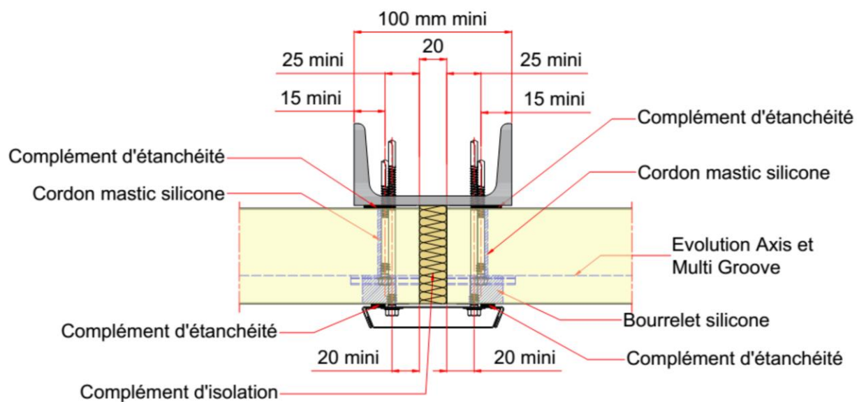
Figure 29 – Exemple d'une jonction verticale en pose horizontale avec panneaux sandwich isolants Evolution Axis ou Multi Groove et 2 fixations traversantes complémentaires par largeur de panneau – Conception 2
