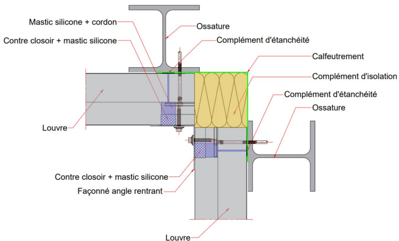
Figure 35 – Exemple d'angle rentrant assemblé sur site en pose horizontale avec panneau sandwich isolant Louvre
