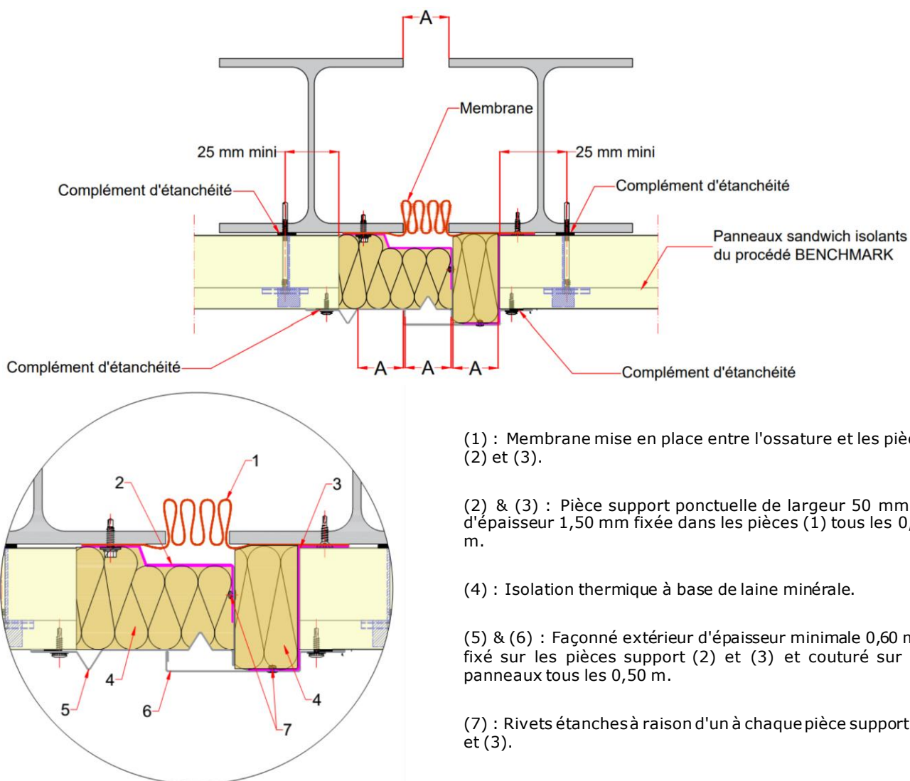
Figure 52 – Exemple d'un joint de dilatation dont le déplacement maximal est de 150 mm avec panneaux sandwich isolants Evolution Axis, Evolution Multi Groove ou Evolution Recess en pose horizontale (hors pose inclinée à fruit positif)
