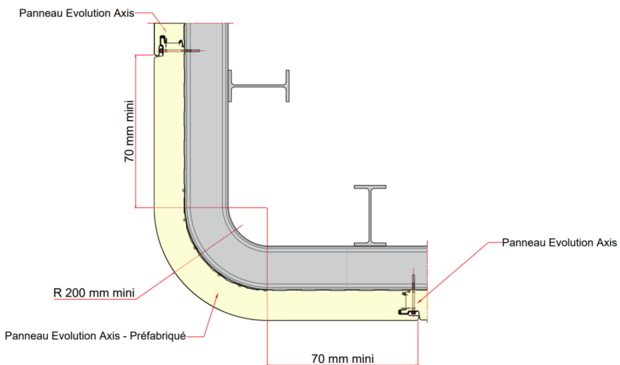
Figure 37 – Exemple d'angle sortant réalisé avec des panneaux préfabriqués cintrés Evolution Axis en pose verticale
