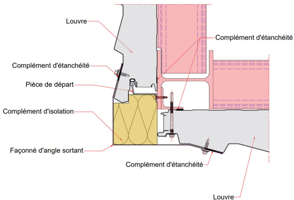
Figure 31 – Exemple d'angle sortant assemblé sur site en pose verticale avec panneau sandwich isolant Louvre
