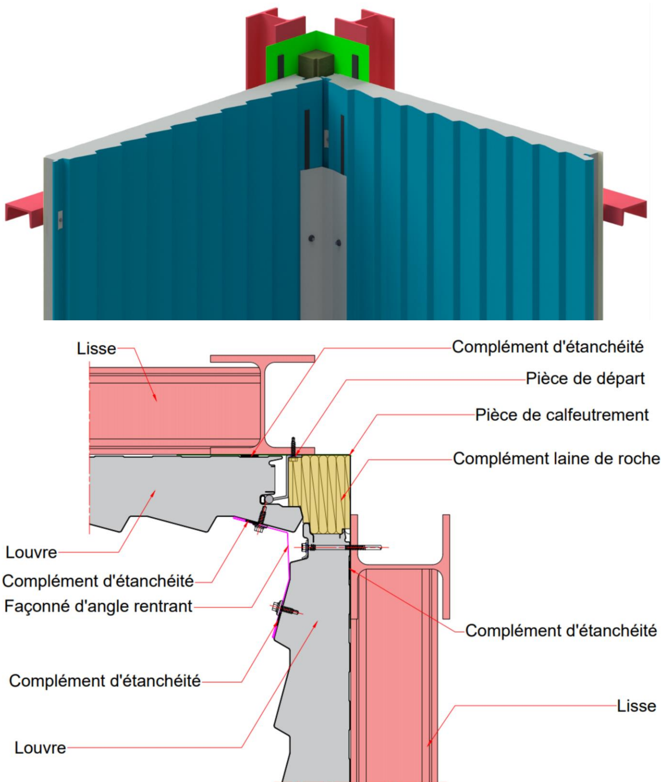
Figure 32 – Exemple d'angle rentrant assemblé sur site en pose verticale avec panneau sandwich isolant Louvre
