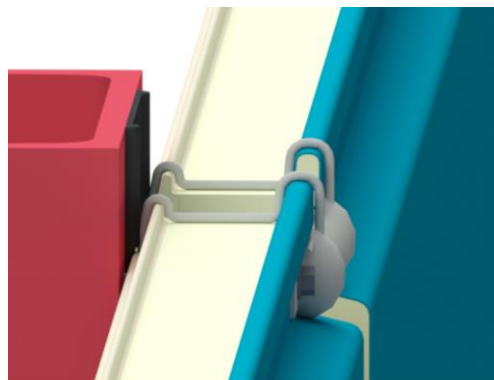
Exemple avec joint EPDM VJ1 ou VJ2 disposé sur appuis
