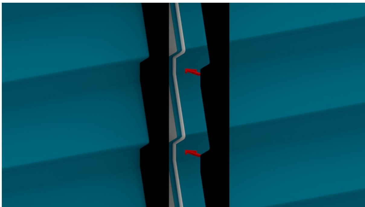
Pose d'un cordon de mastic silicone avant mise en place du contre closoir
