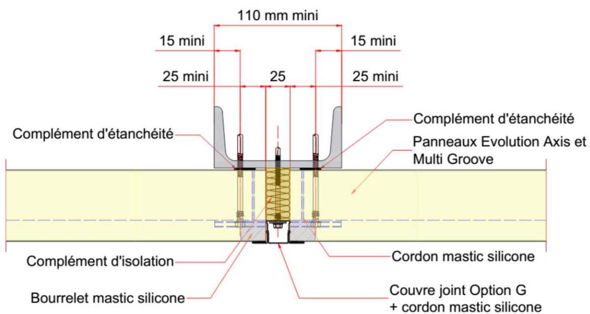
Figure 23 – Exemple d'une jonction verticale en pose horizontale avec panneaux sandwich isolants Evolution Axis ou Multi Groove et couvre-joint option G (Affleurant) sur ossature acier
