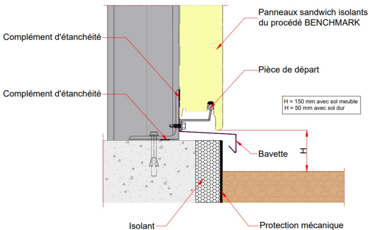
Figure 15 bis – Bas de bardage en pose horizontale sur longrine
