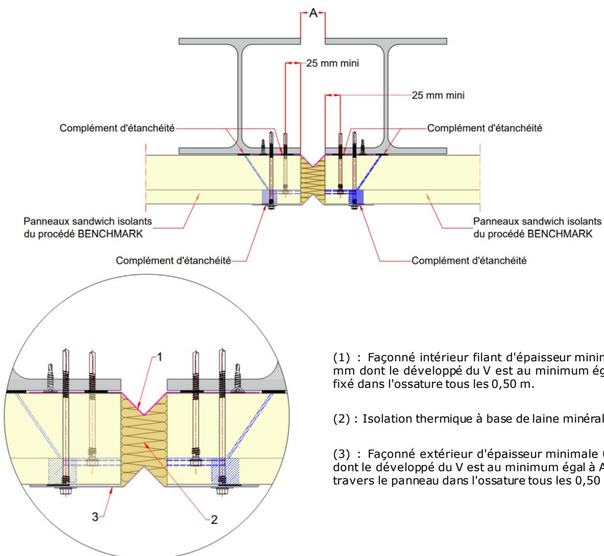
Figure 51 – Exemple d'un joint de dilatation dont le déplacement maximal est de 50 mm avec panneaux sandwich isolants Evolution Axis, Evolution Multi Groove ou Evolution Recess en pose horizontale
