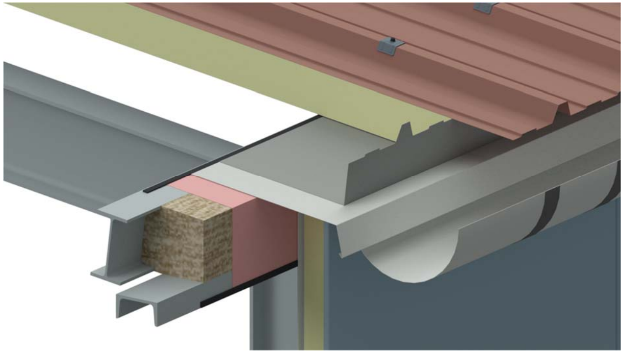
Figure 11 – Egout avec gouttière pendante
