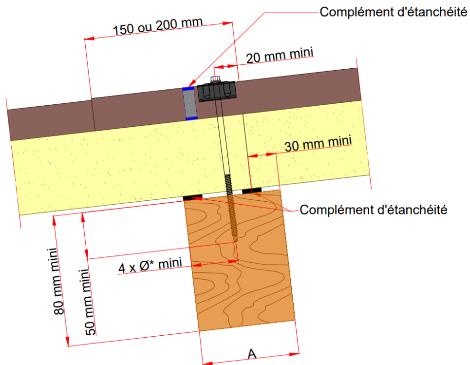
Figure 5 ter – Dispositions au droit d'un appui bois recevant un recouvrement transversal
