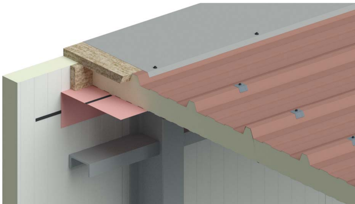
Figure 15 – Rive contre pignon
