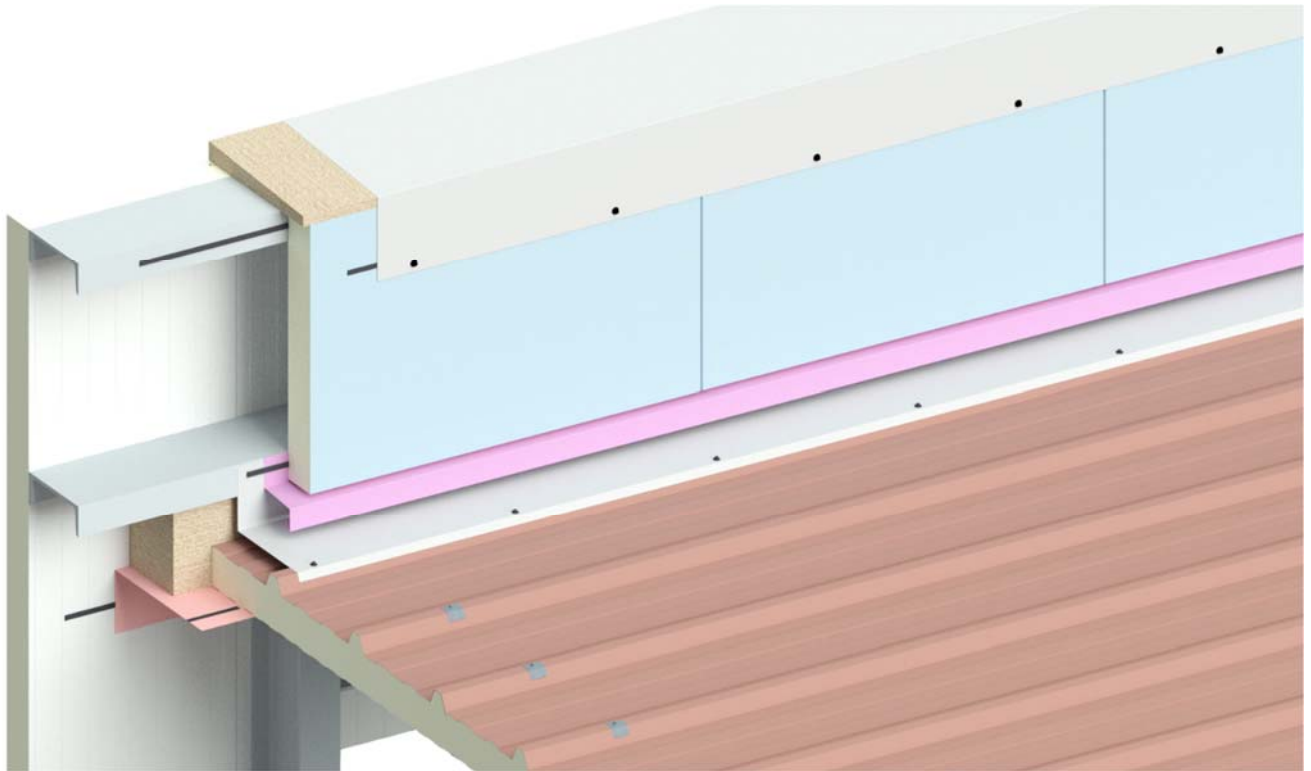
Figure 16 – Rive contre acrotère
