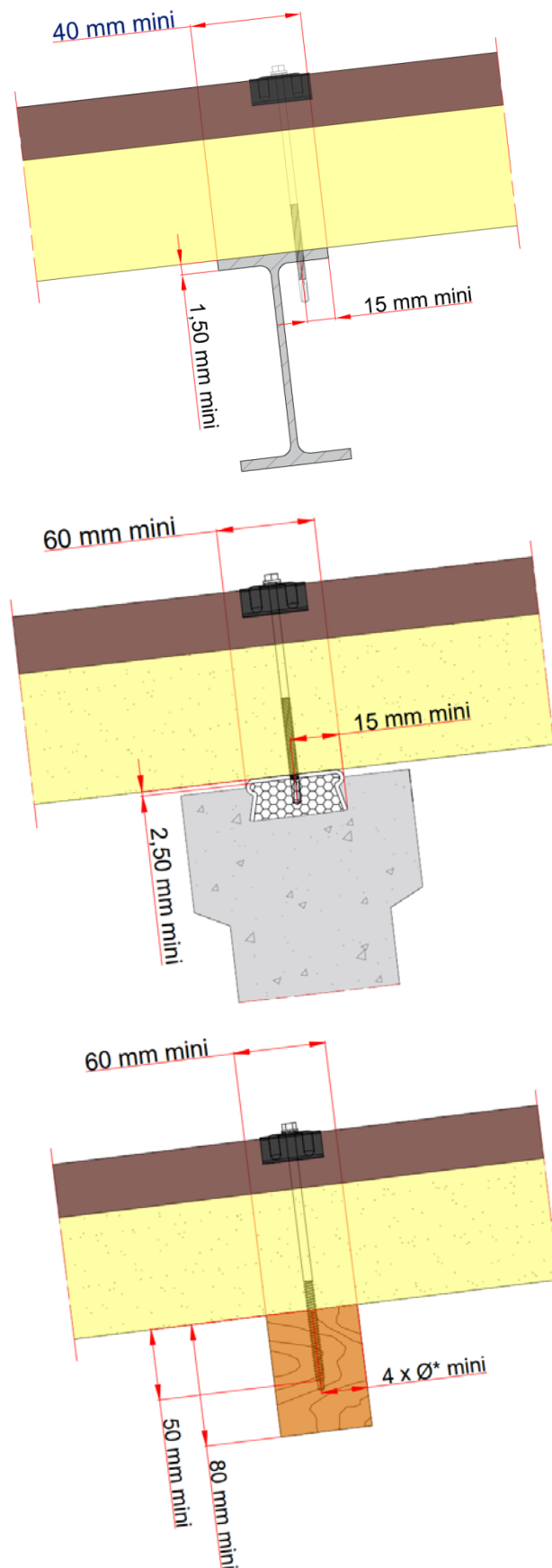
Figure 4 – Largeur minimale des appuis intermédiaires
