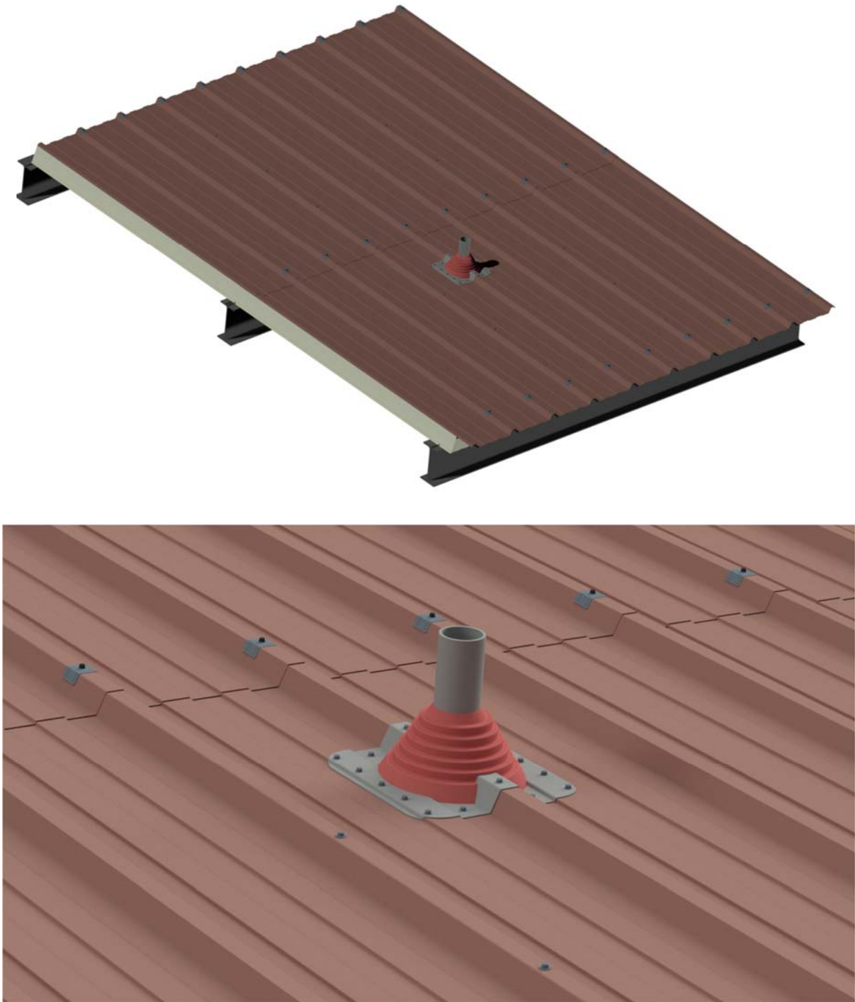
Figure 17 – Pénétration avec manchon d'étanchéité caoutchouc
