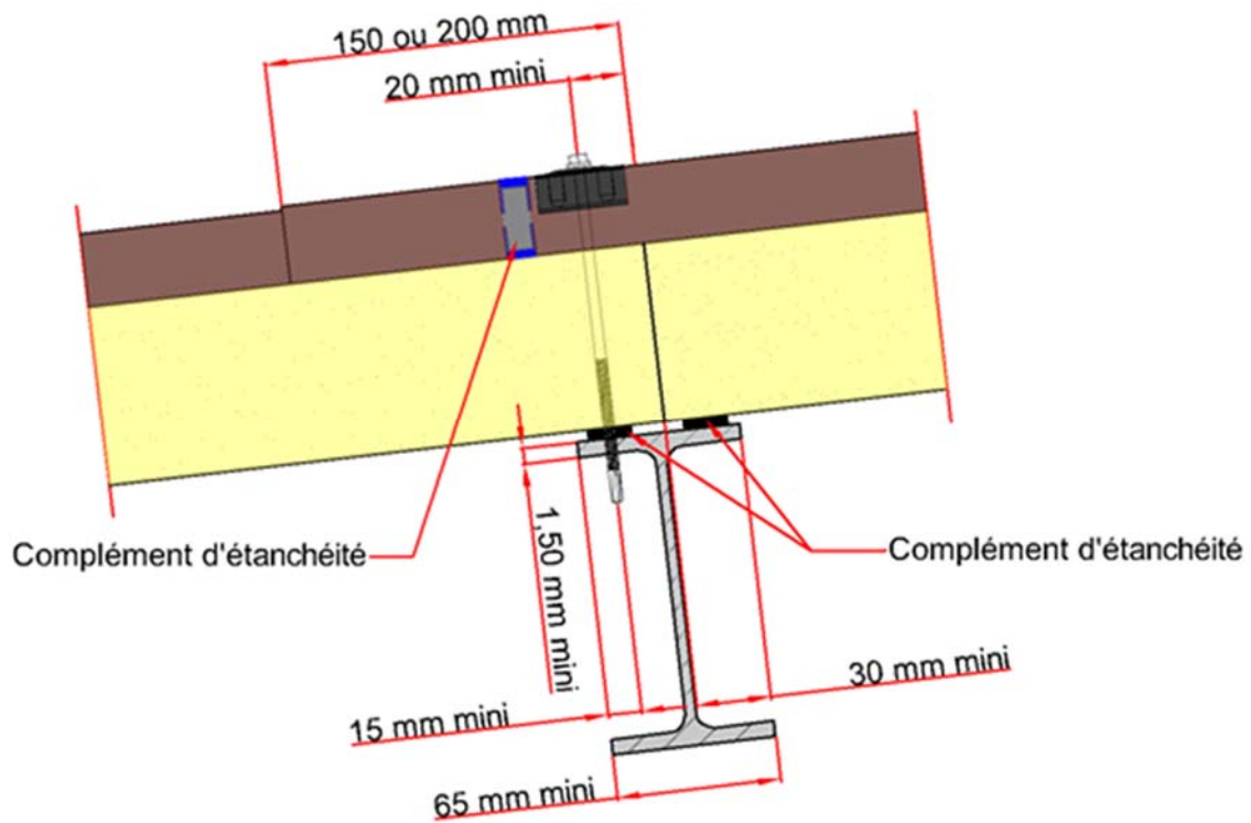
Figure 5 – Dispositions au droit d'un appui acier recevant un recouvrement transversal
