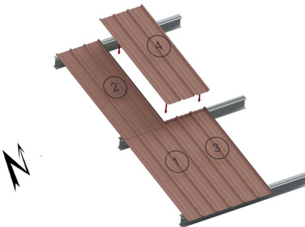
Panneaux type gauche
