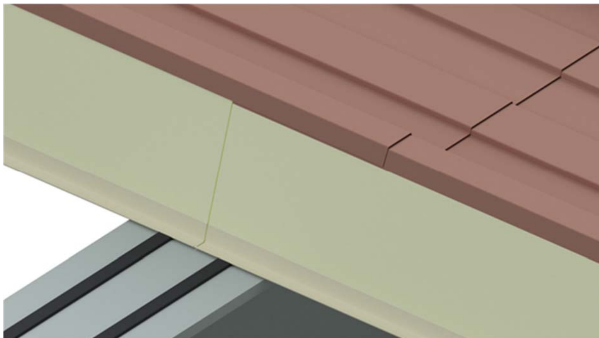
Figure 6 Ter – Dispositions au niveau des joints sur appuis pour les locaux à faible et moyenne hygrométrie dont la température intérieure est supérieure à 12°C.
