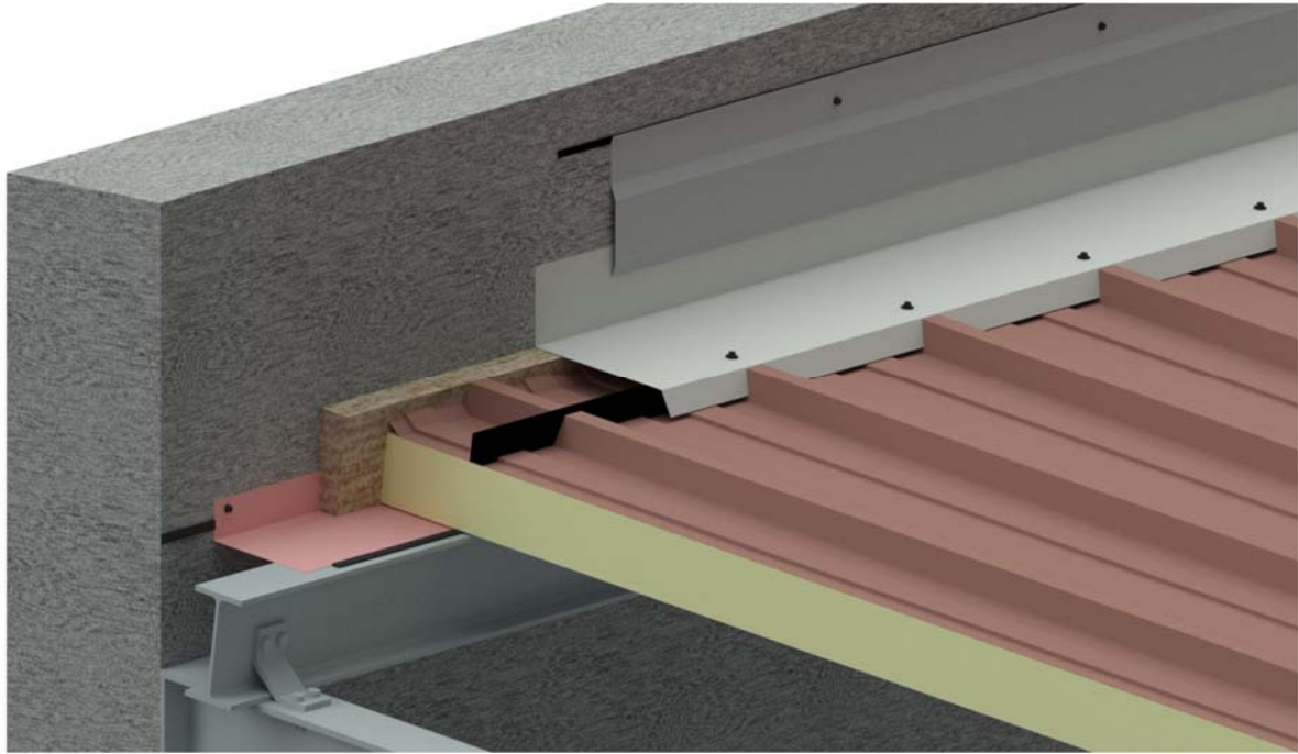
Figure 10 – Faitage en solin contre mur
