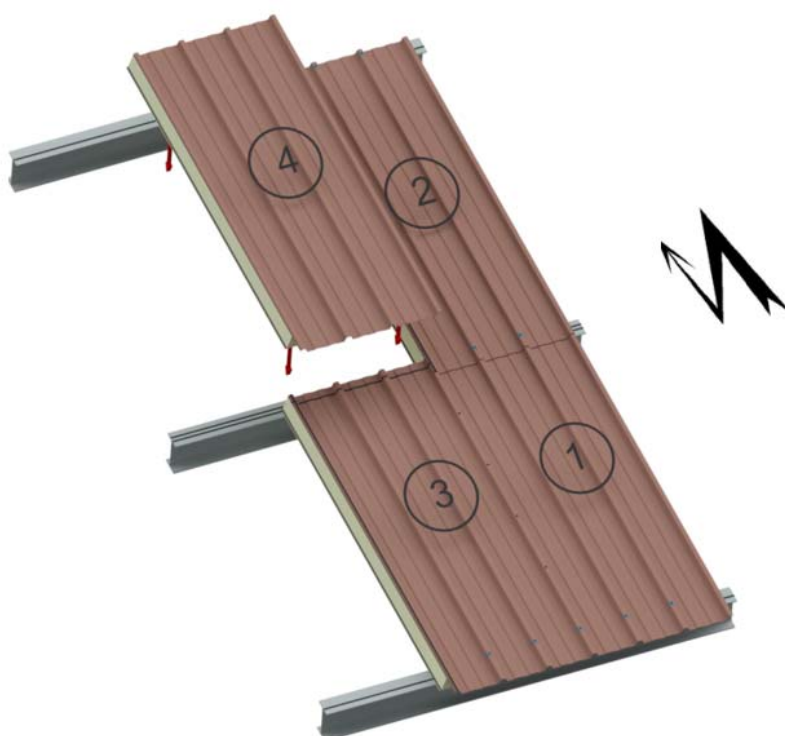
Panneaux type droit
