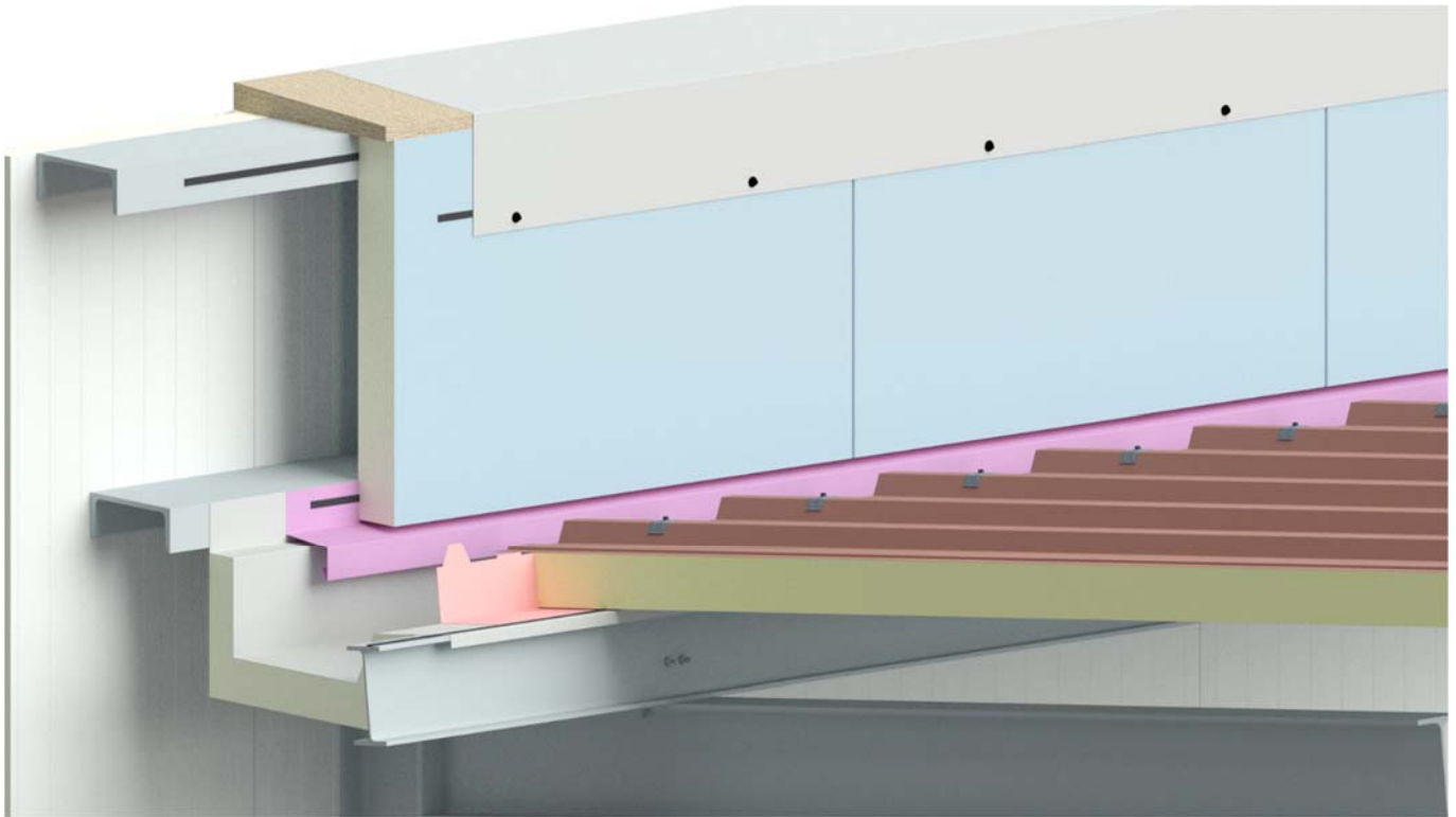
Figure 14 – Chéneau contre acrotère
