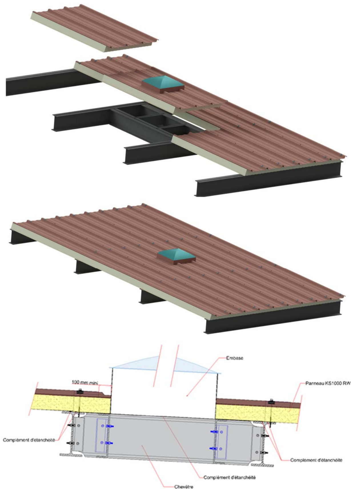
Figure 18 – Pénétration avec embase polyester isolée
