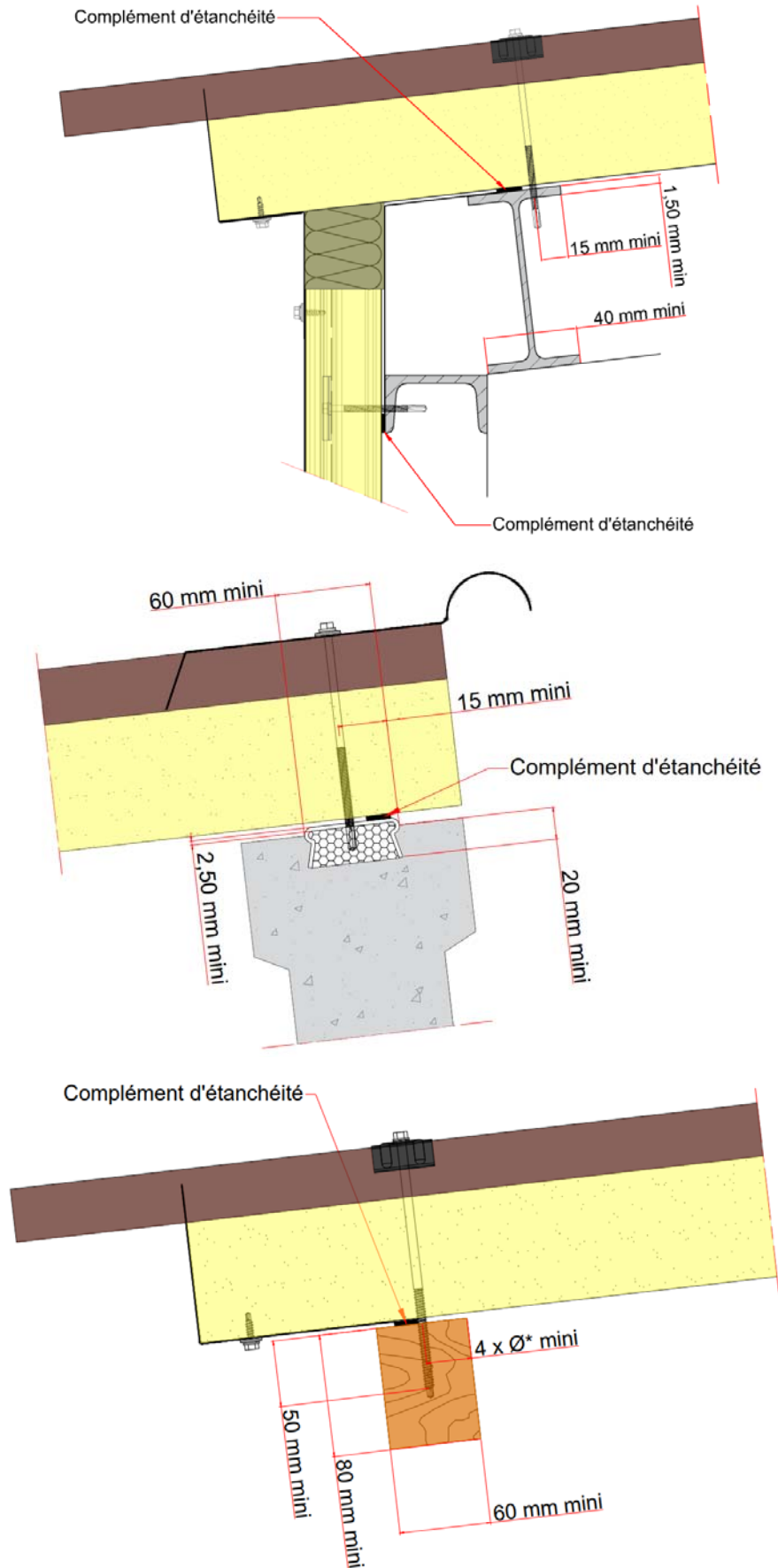
Figure 3 – Largeur minimale des appuis d'extrémité
