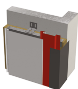
Jonction à un mur existant
