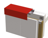
Haut de bardage / Couvertine d'acrotère
