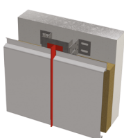
Jonction entre lames / à aiguille
