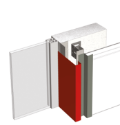
Ouverture / Jambage à joint creux
