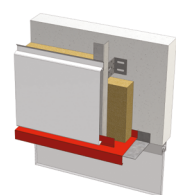
Ouverture / Linteau horizontal
