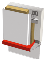
Ouverture / Appui de rive et linteau vertical
