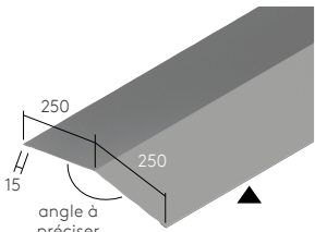
Sous-faîtière
