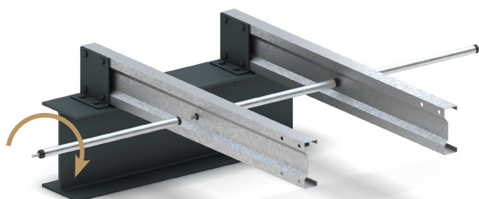
Assemblage des liernes par vissage
