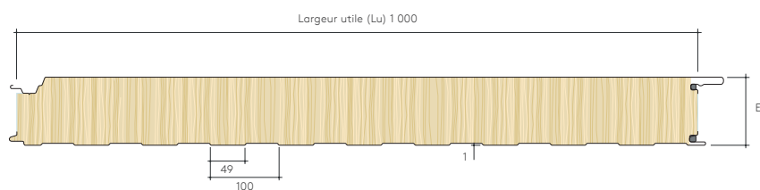
Profil lisse
