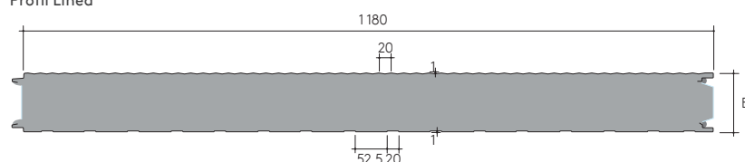
Profil Linéa
