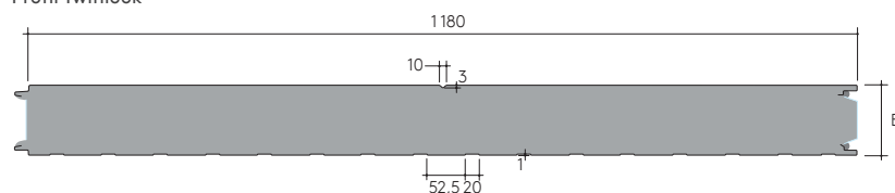
Profil Twinlook
