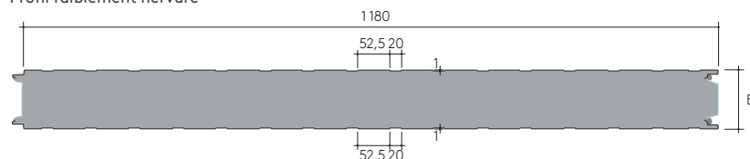
Profil faiblement nervuré
