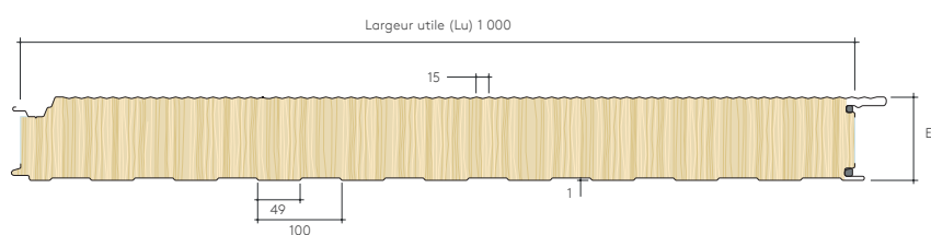
Profil micro-nervuré
