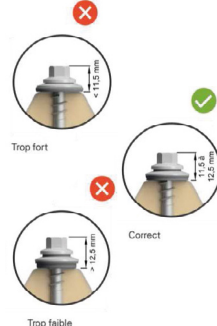
SFS SOK-IT®-PLUS - Butée de profondeur
