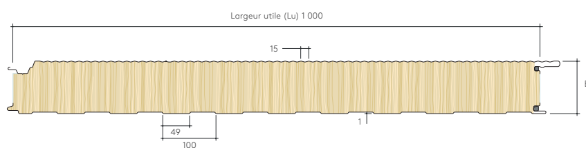
Profil micro-nervuré
