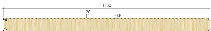
Profil Linéa
