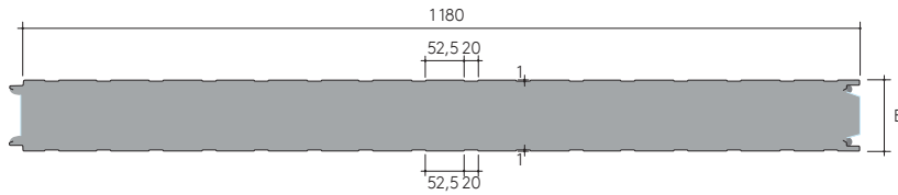
Profil faiblement nervuré
