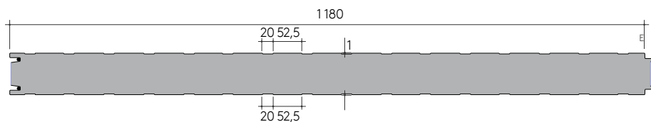
Profil Linéa
