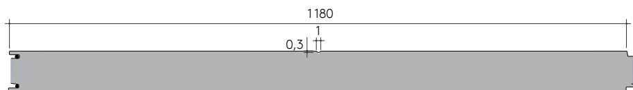
Profil Twinlook
