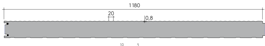
Profil Twinlook
