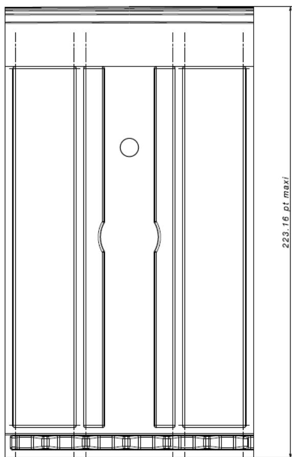
Figure 19 : Plan Réhausse 45 polymère
