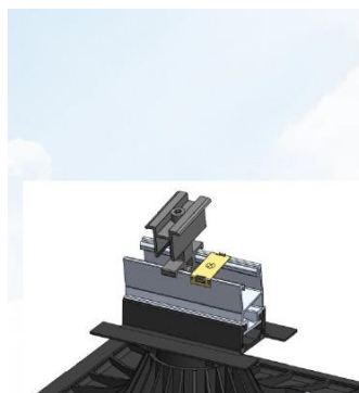
Installer une Terragrif par réhausse 45 (basse)
