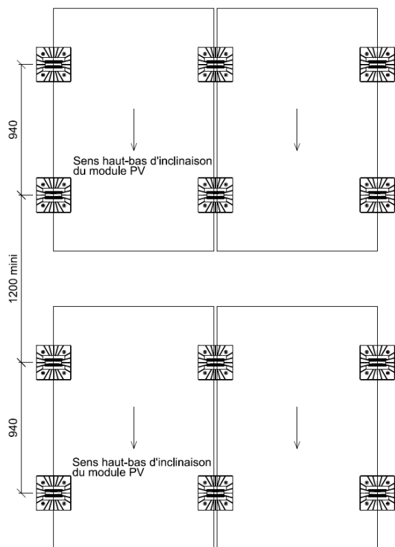
Figure 30 : Implantation des plots SOPRASOLAR FIX EVO PVC/TPO avec modules photovoltaïques en inclinaison simple shed - réhausse polymère
