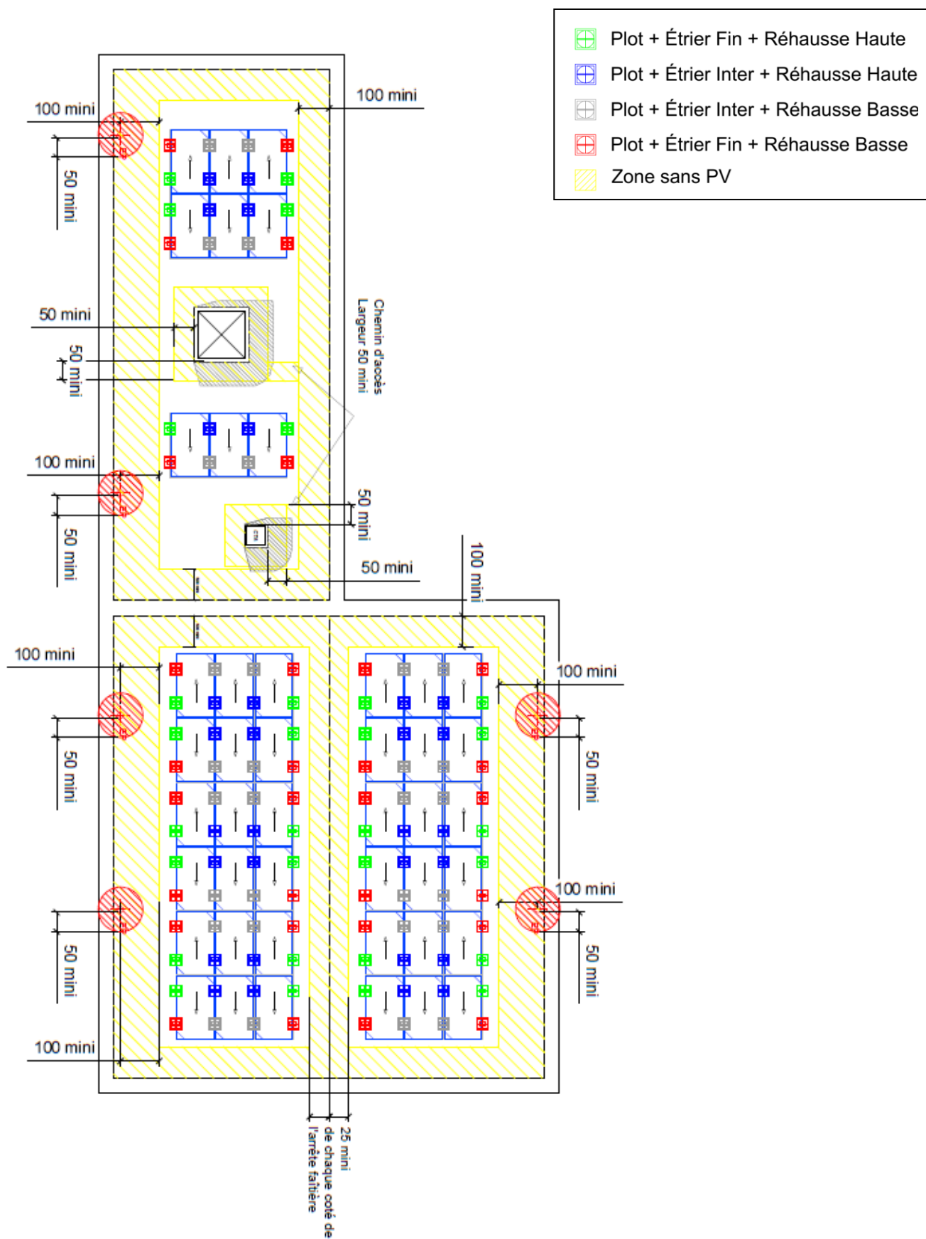
Figure 42 : Exemple calepinage et préparation de la toiture avec modules photovoltaïques inclinés en orientation « double Shed»
