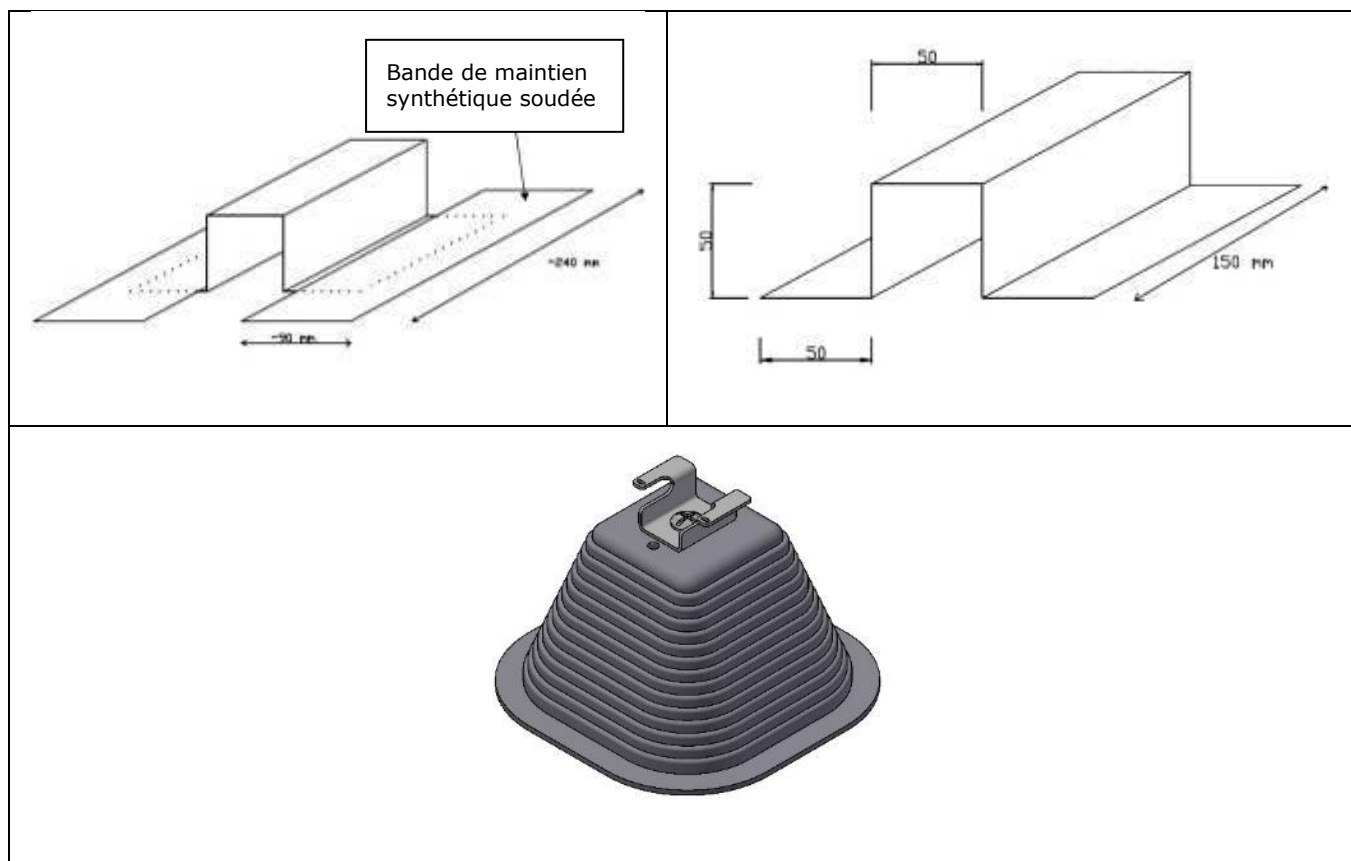
Figure 21 : Supports de chemin de câble
