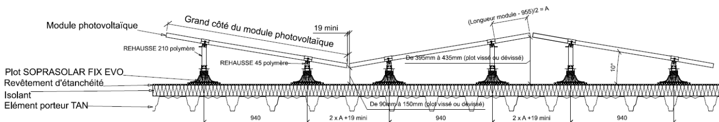
Figure 9 : Vue en coupe (dans le sens de la longueur des modules) du procédé avec modules photovoltaïques de longueur 1755mm en inclinaison simple shed-réhausse polymère
