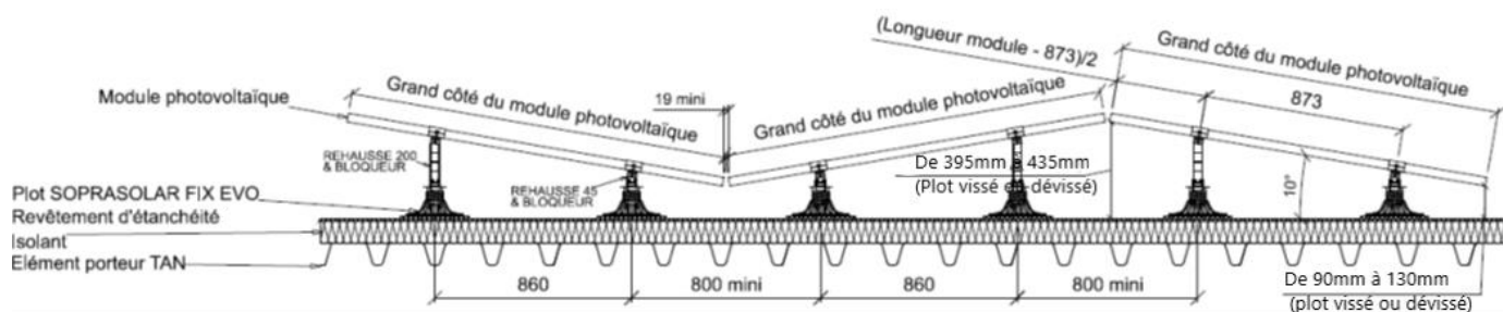
Figure 6 : Vue en coupe (dans le sens de la longueur des modules) du procédé avec modules photovoltaïques de longueur 1755mm en inclinaison double shed-réhausse aluminium
