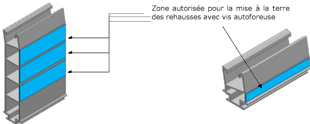
Localisation zone de perçage pour mise à la terre des rehausses Aluminium par vis autoperceuse (mise à la terre de la rehausse 200 aluminium uniquement)
