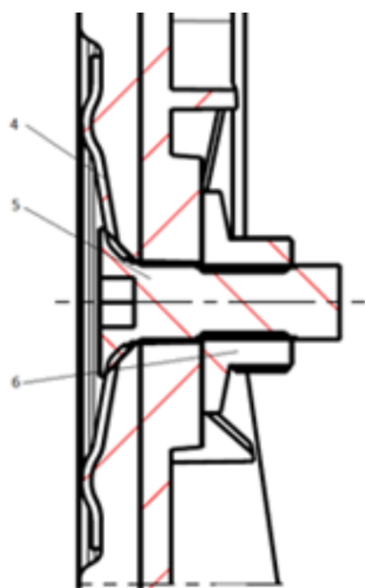
Coupe sur la visserie
