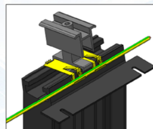
Insérer le câble Vert/Jaune dans la gorge H07VK6 V/J UNIQUEMENT
