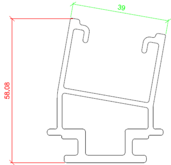
Figure 1 : Plan Réhausse 45 aluminium
