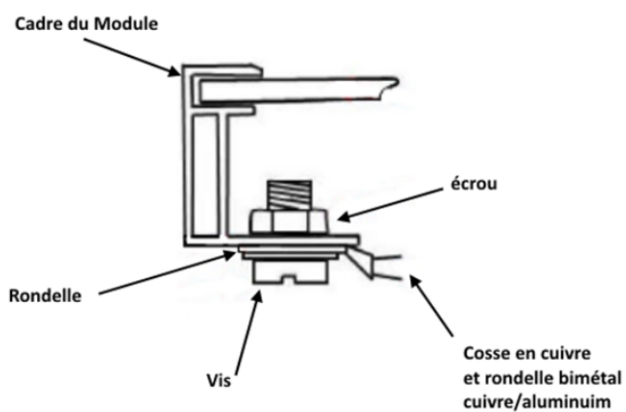
Figure 26 – Mise à la terre du module
