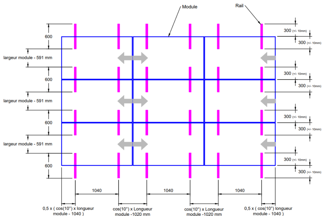
Figure 37 - Implantation des ensembles « Rail » / modules inclinées double shed
