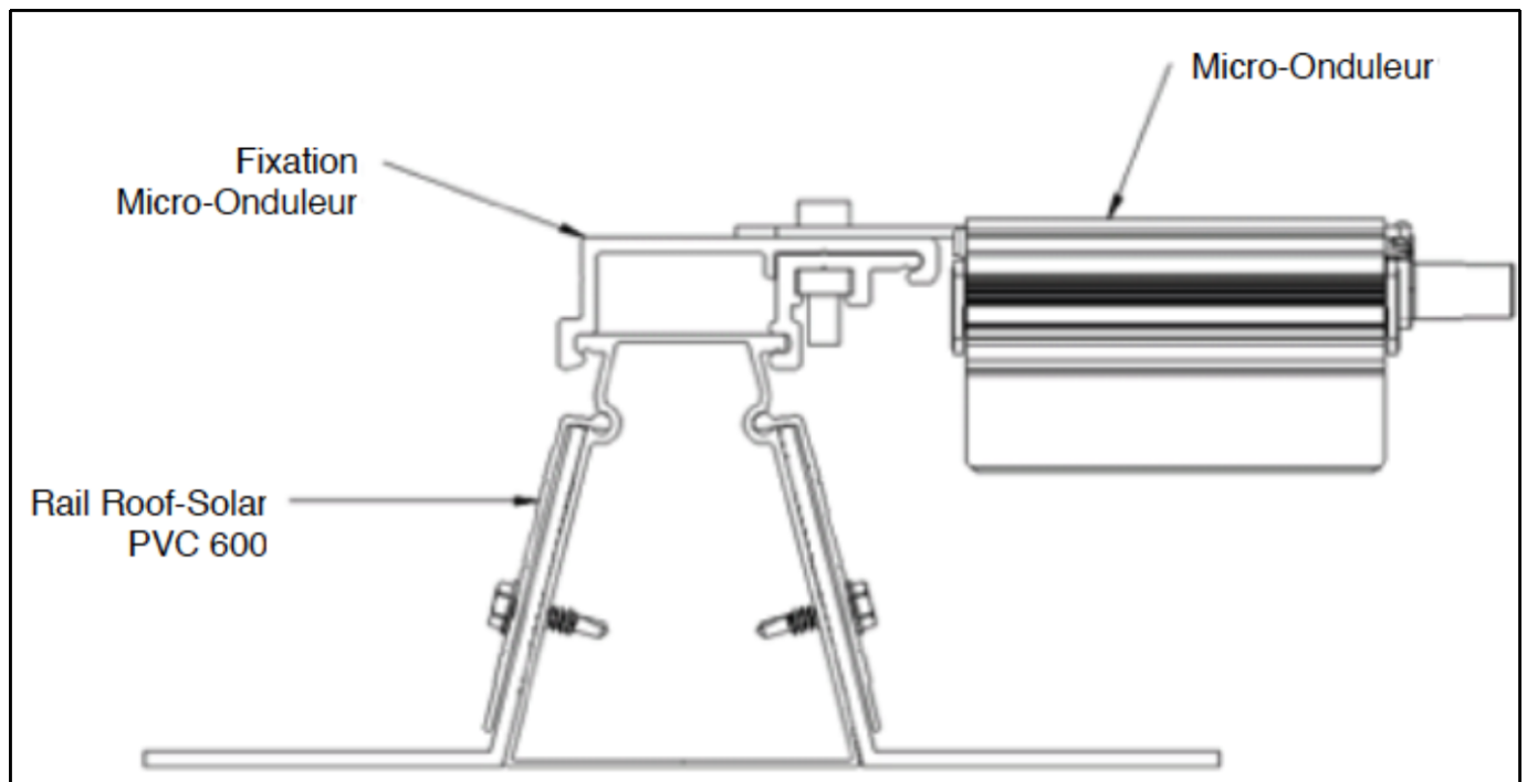
Figure 27 – Micro-onduleur
