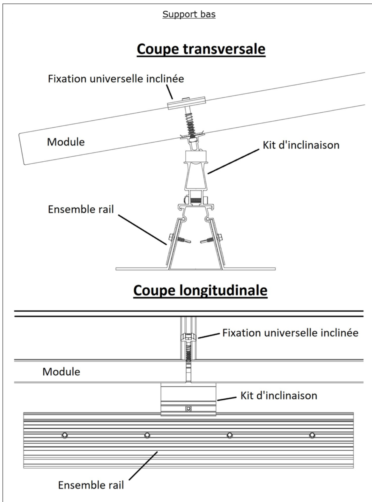
Figure 33 (suite) - Assemblage rail / kit d'inclinaison / module
