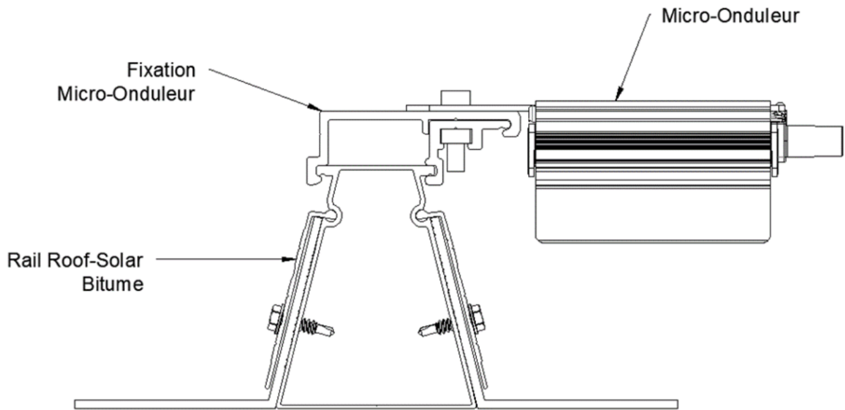
Figure 26 - Micro-onduleurs
