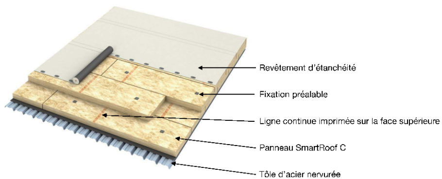
Figure 21 - Sens de pose des panneaux SmartRoof C
