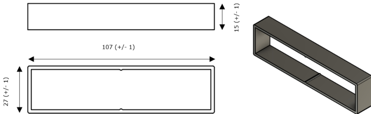
Figure 20 - Cale rotule du kit d'inclinaison du procédé ROOF-SOLAR BITUME TAN DTU – Plat & Incliné
