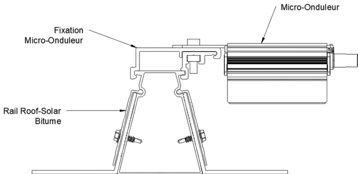
Figure 24 - Micro-onduleurs
