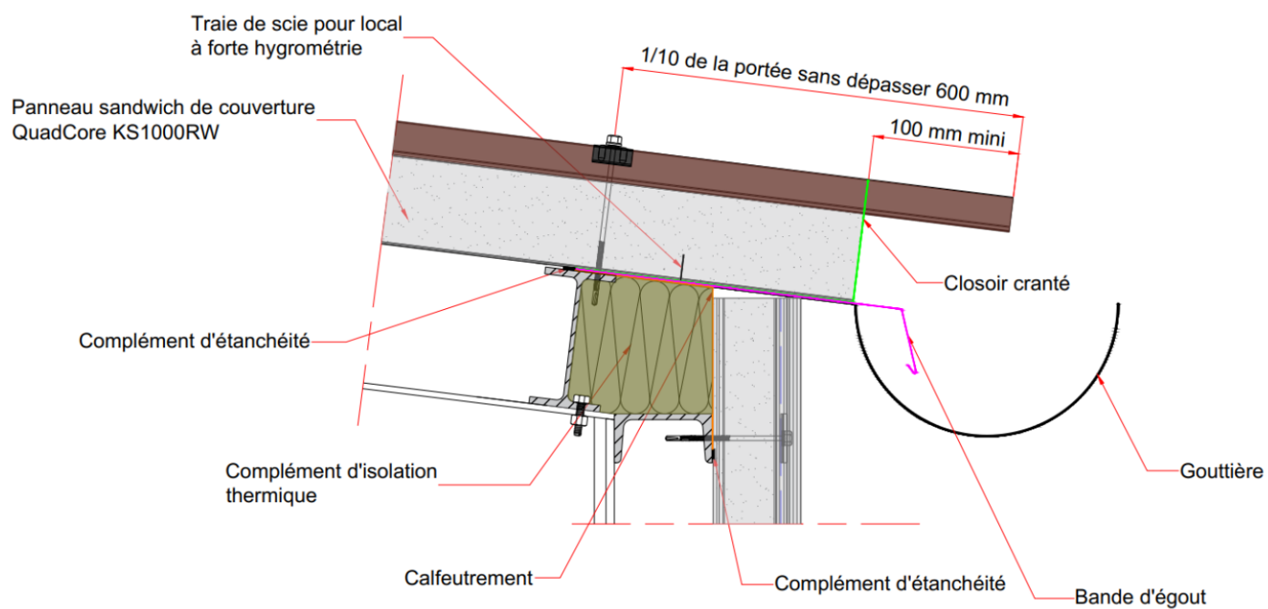
Figure 11 – Egout avec gouttière pendante
