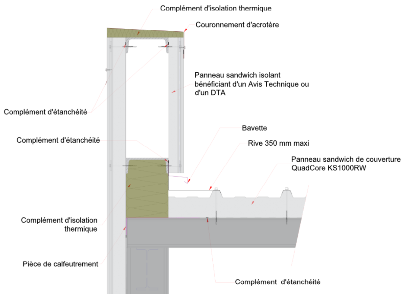
Figure 16 – Rive contre acrotère
