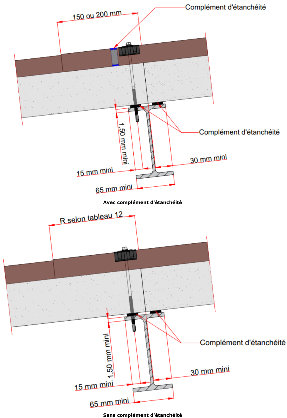
Figure 5 – Dispositions au droit d'un appui acier recevant un recouvrement transversal
