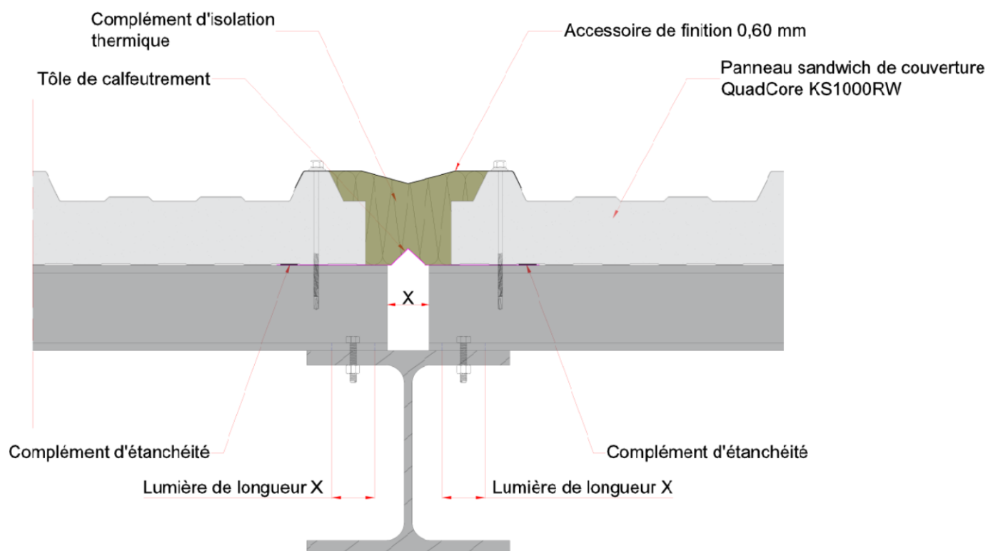
Figure 19 – Joint de dilatation (déplacement maxi de 50 mm)
