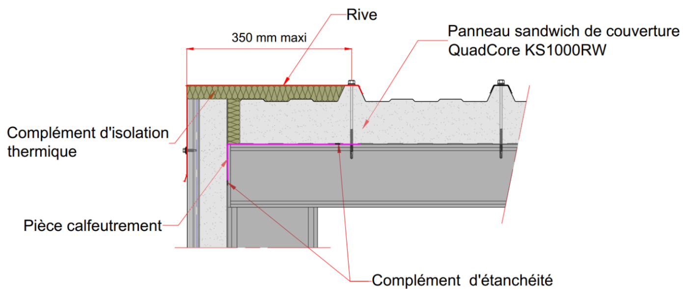
Figure 15 – Rive contre pignon
