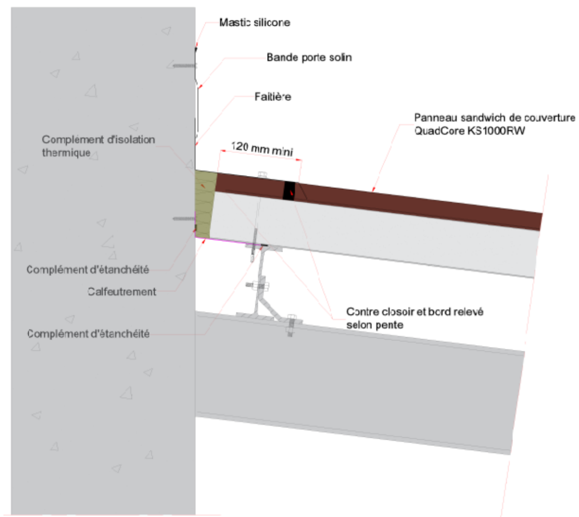
Figure 10 – Faitage en solin contre mur
