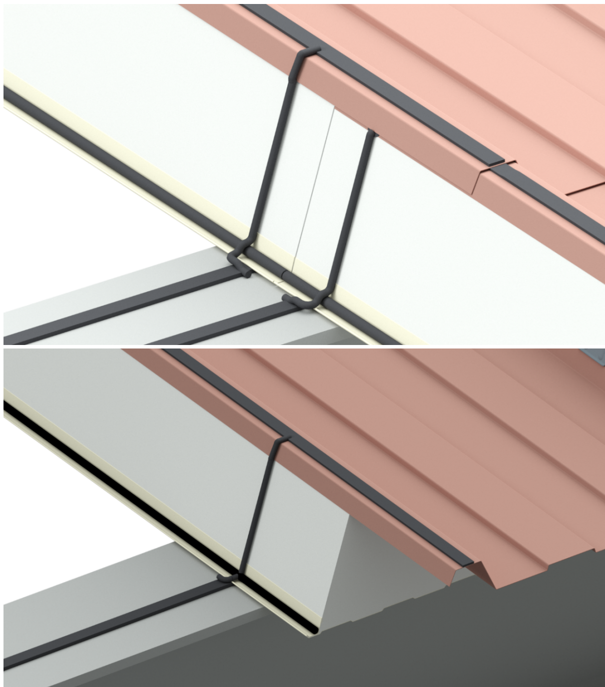
Figure 6 – Principe de raccordement entre les compléments d'étanchéité longitudinaux et les joints d'étanchéité sur appuis pour les locaux climatisés avec pression de vapeur compris entre 5 et 10 mm Hg situés en climat de plaine et/ou pour tous les locaux situés en climat de montagne.
