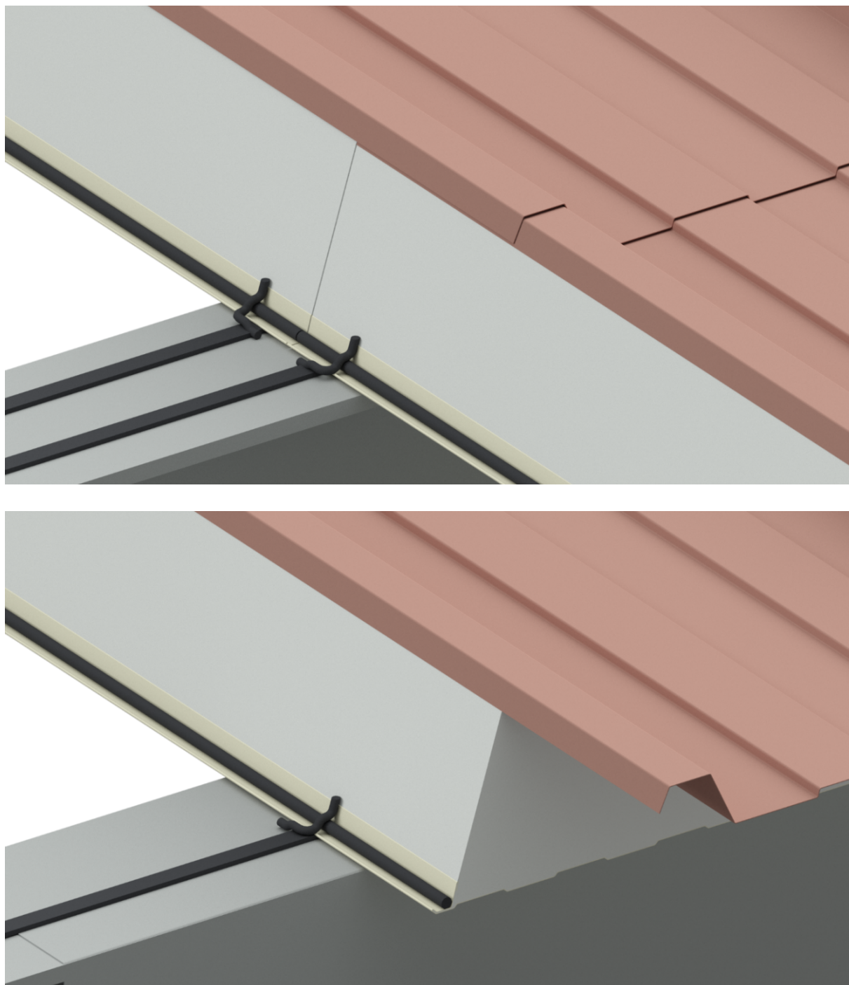
Figure 6 Bis – Principe de raccordement entre les compléments d'étanchéité longitudinaux et les joints d'étanchéité sur appuis en l'absence de complément d'étanchéité longitudinal extérieur pour les locaux :
