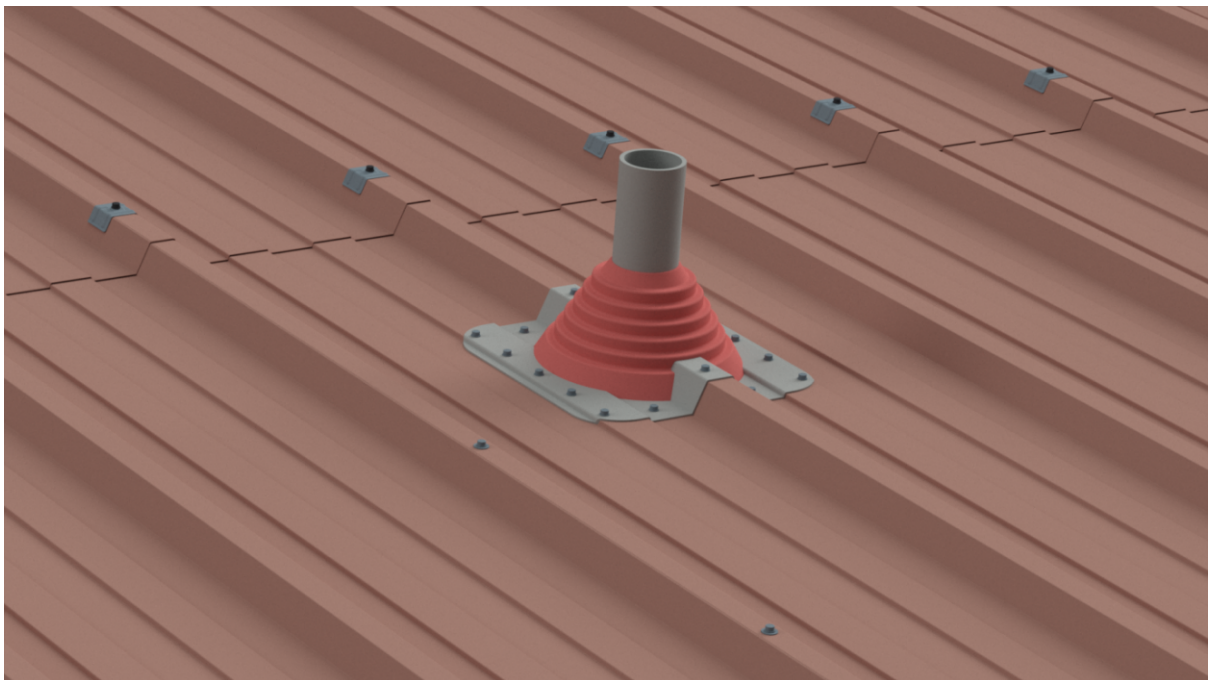
Figure 17 – Pénétration avec manchon d'étanchéité caoutchouc
