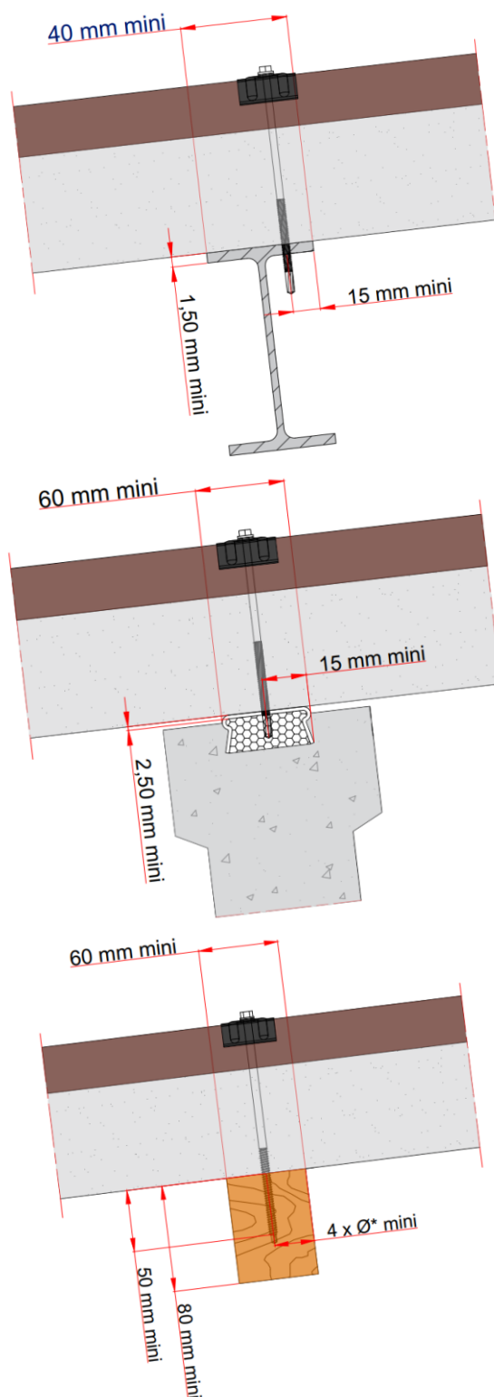
Figure 4 – Largeur minimale des appuis intermédiaires
