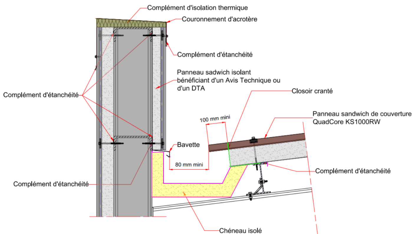
Figure 14 – Chéneau contre acrotère
