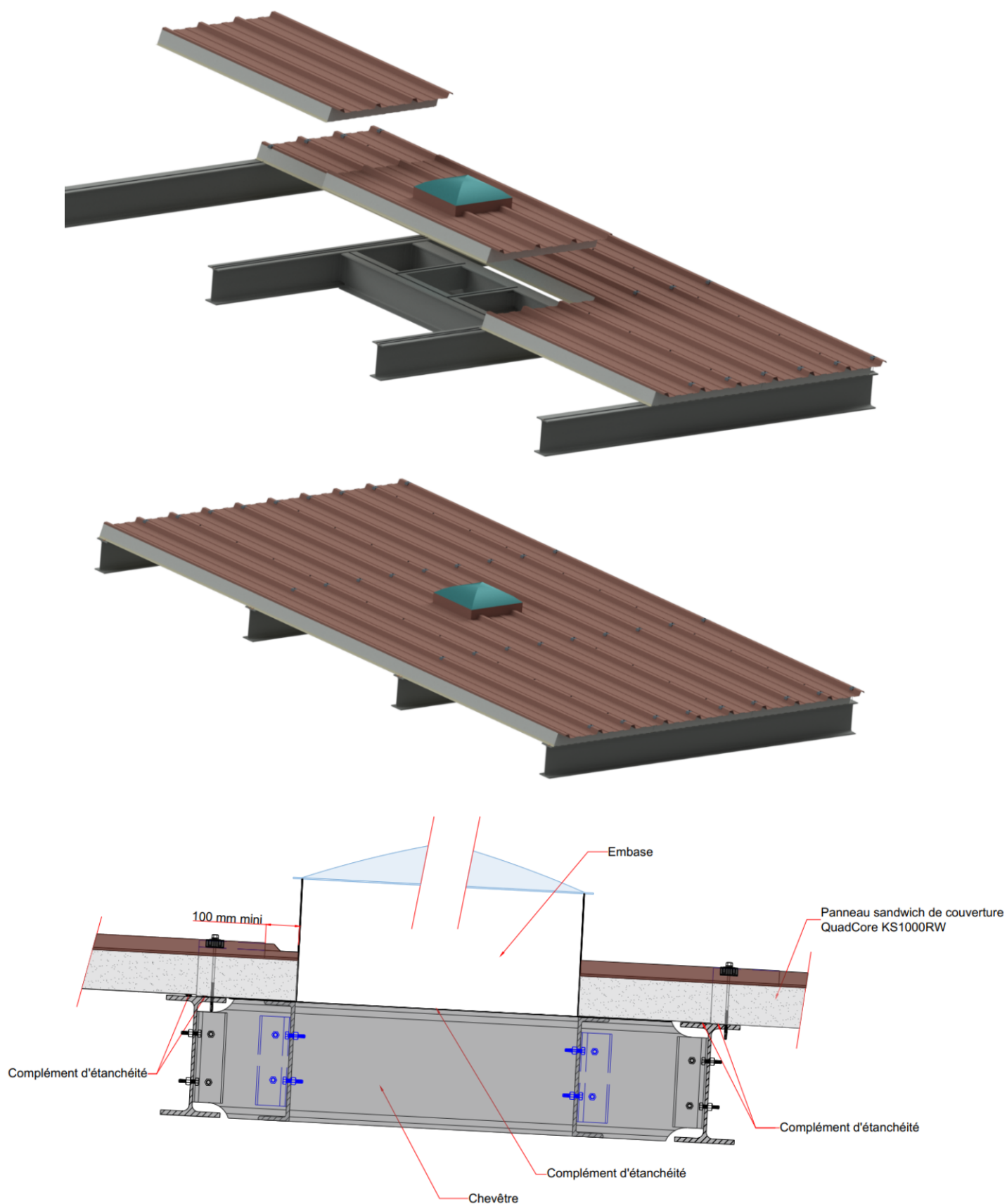
Figure 18 – Pénétration avec embase polyester isolée
