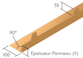
Closoir cranté
