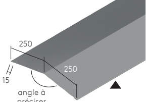
Sous-faîtière
