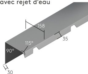
Bandeau de faîtage crantée avec rejet d'eau
