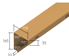
Faîtière simple crantée
