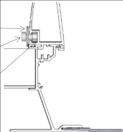
Fixation de la rehausse Tilt GC FE basse sur l'ossatures support
