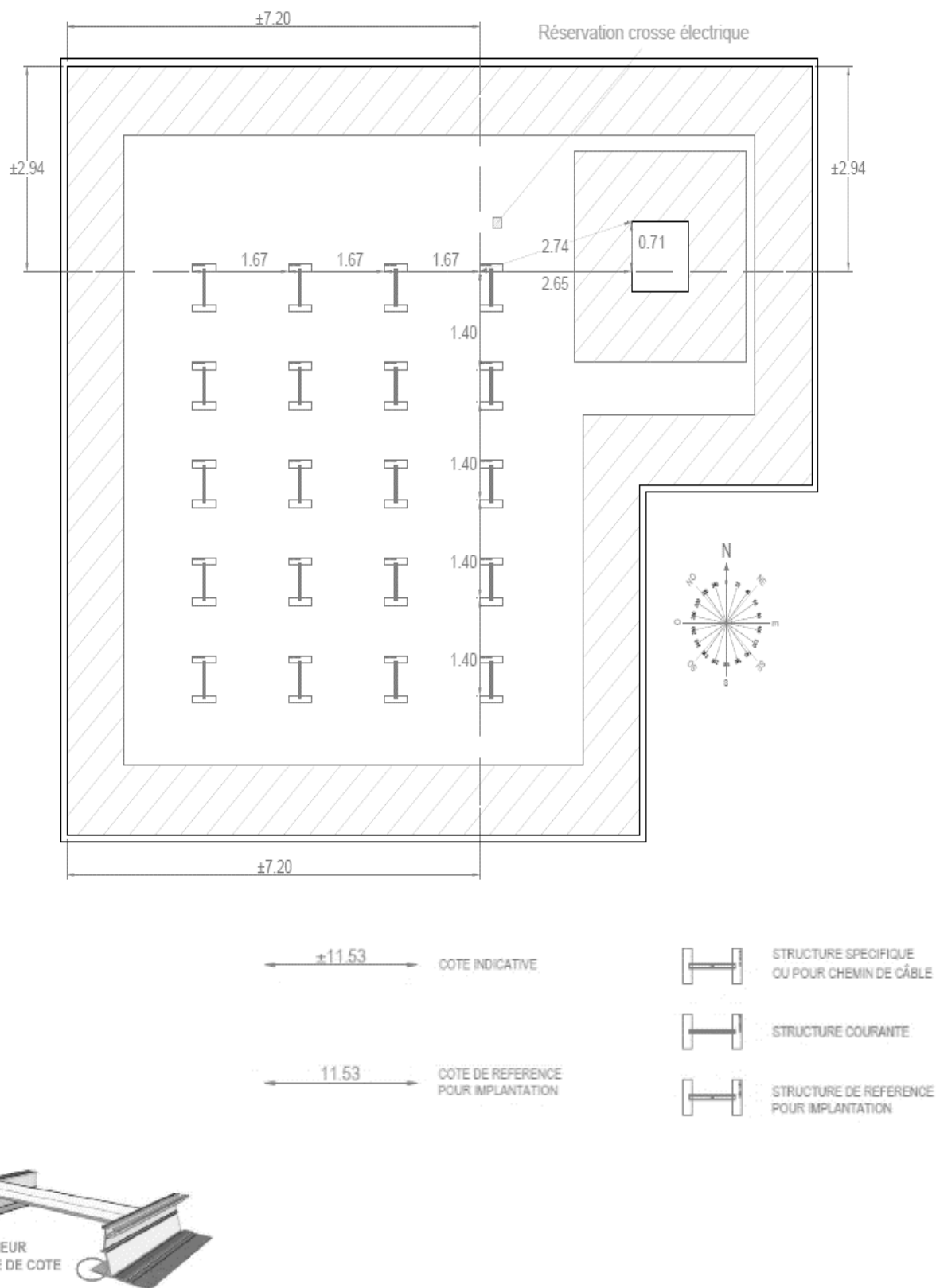
Figure 18 – Exemple de plan d'implantation des ossatures supports iNova PV Lite
