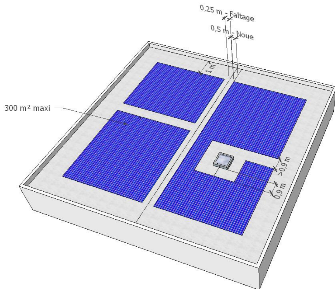
Figure 16 – Principe d'implantation des champs photovoltaïques
