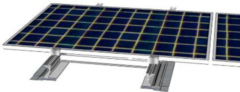
Figure 19 – Mise en oeuvre des modules à plat
