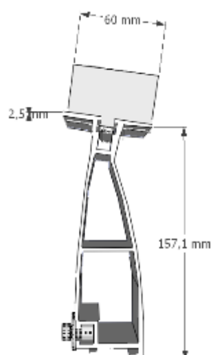
Figure 7 – Rehausse Tilt GC FE basse de 8°
