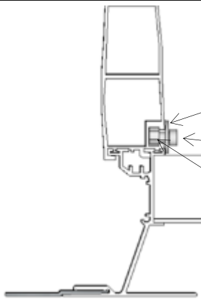
Fixation de la rehausse Tilt GC FE haute sur l'ossatures support
