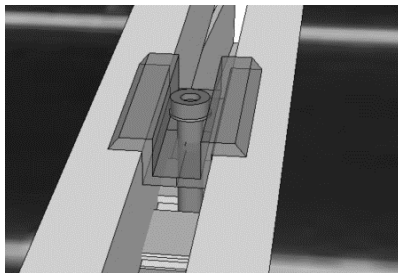
Mise en place de la bride centrale : Vis M8X (suivant cadre)+ Rondelle + Ecrou carré dans la gorge de la rehausse
