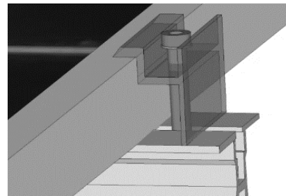
Mise en place de la bride Latérale : Vis M X (suivant cadre) + Rondelle + Ecrou carré dans la gorge de la rehausse
