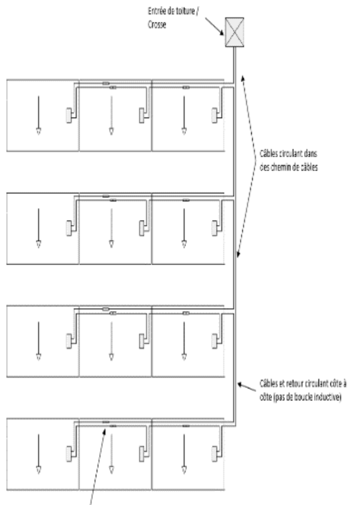
Figure 9 – Exemple de plan de cablage des modules photovoltaïques et maintien des câbles
