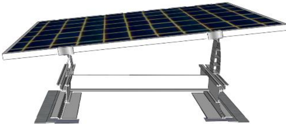
Ossature support iNova PV Lite Tilt GC FE PVC-FPO 40 E 87 avec module photovoltaïque monté
