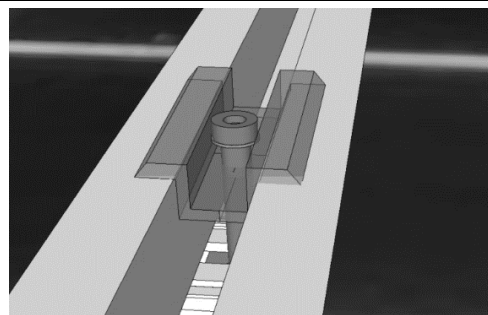
Ossature support Susncape iNova PV Lite 40 E 87 avec module photovoltaïque monté
