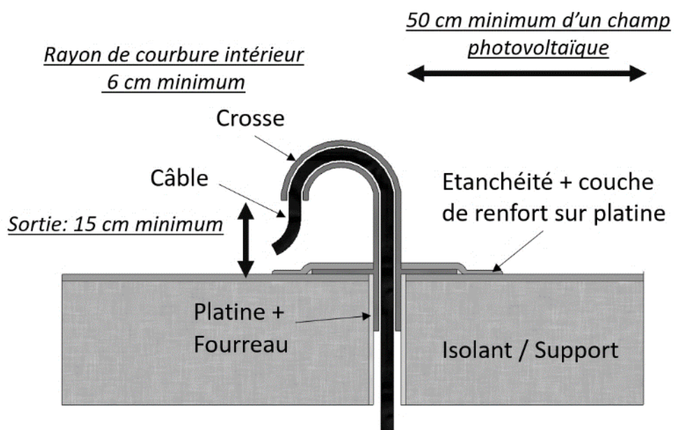
Figure 15 – Crosse de passage de câble
