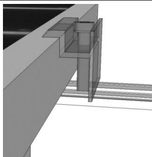
Ossature support Susncape iNova PV Lite 40 E 87 avec module photovoltaïque monté
