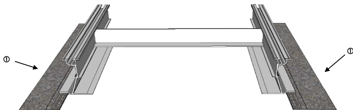
Figure 20 – Positionnement des bandes de raccordement Parafor iNova (§ 1.4.3.2.4 et § 1.10.5.3.3)
