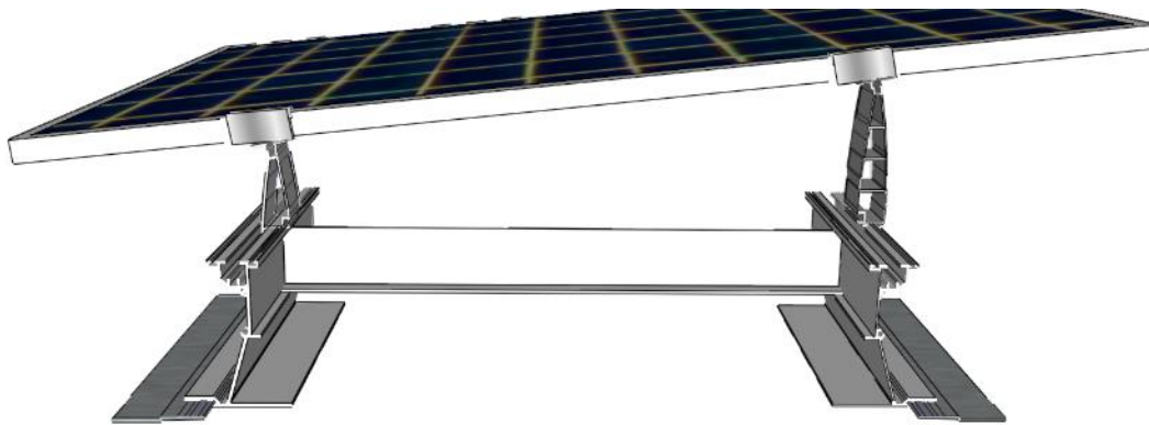
Figure 22 – Mise en oeuvre des modules en version inclinée
