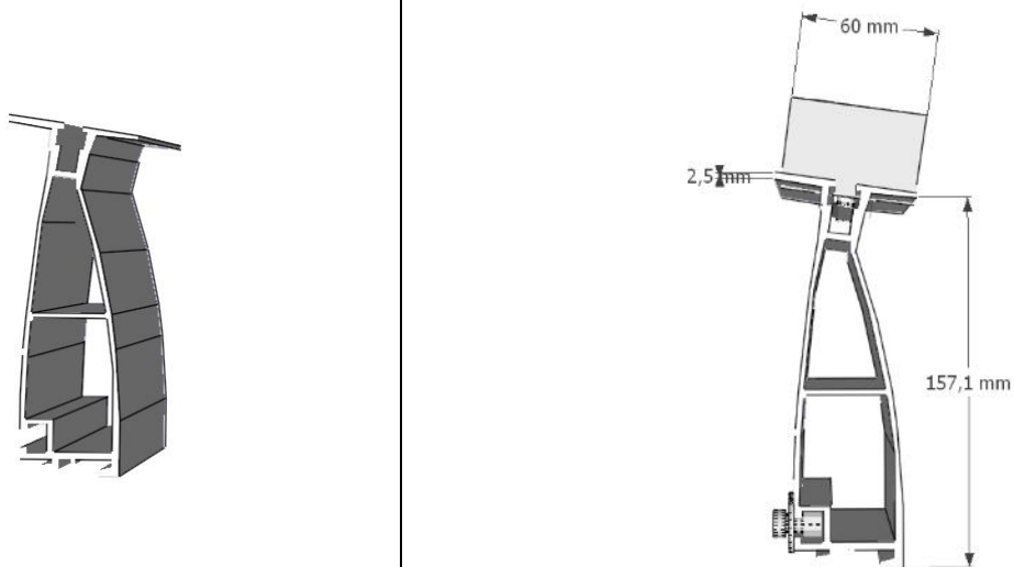
Figure 7 – Rehausse Tilt GC FE basse de 8°
