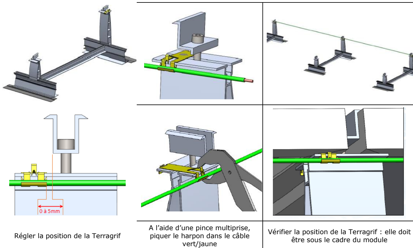
Figure 11 – Mise à la terre des modules et des ossatures supports iNova PV Lite avec la TerraGrif TM de Mobasolar (référence : RL0.6 x 20 x 60) – Version inclinée
