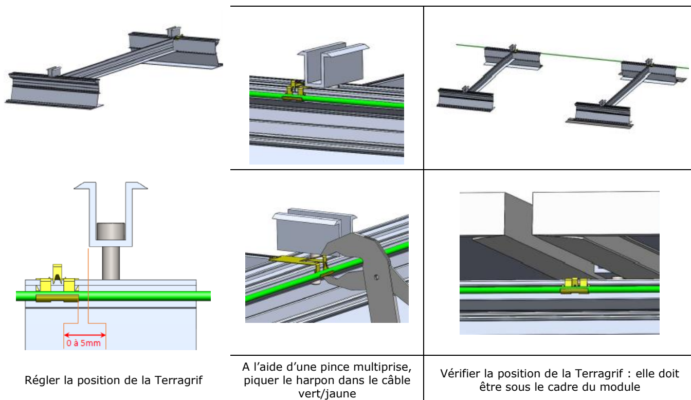
Figure 12 – Mise à la terre des modules et des ossatures supports iNova PV Lite avec la TerraGrif TM de Mobasolar (référence : RL0.6 x 20 x 44) – Version à plat
