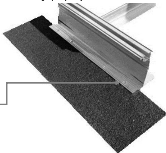
Détail de l'assemblage de l'entretoise
