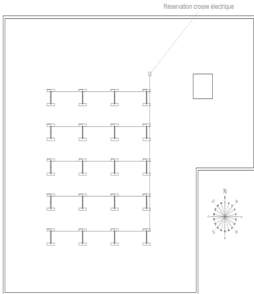
Figure 13 – Exemple de câblage de la mise à la terre
