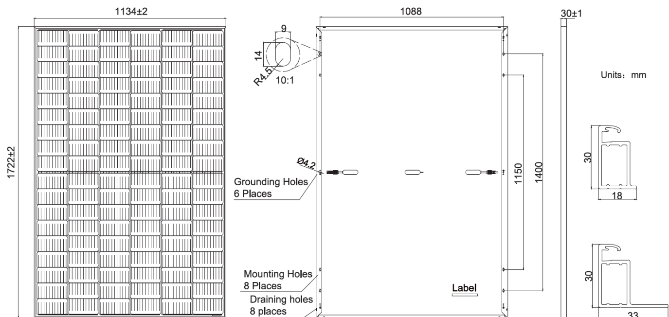
Module photovoltaïque JAM54S30/MR / JAM54S31/MR, et cadre
