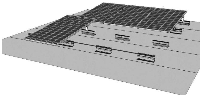
Figure 14 – Mise à la terre des ossatures support iNova PV Lite
