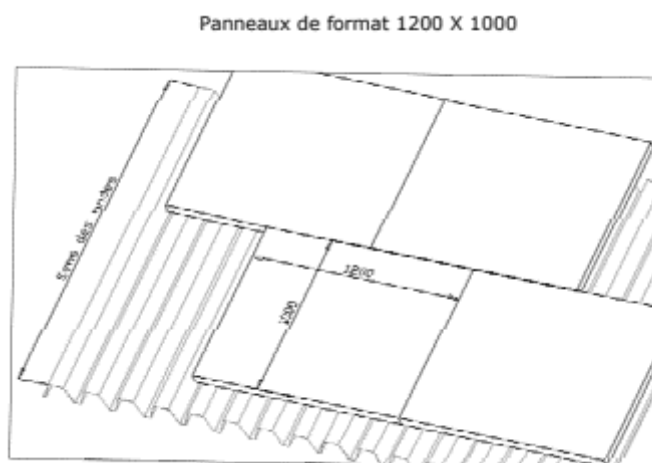
Figure 27– Mise en œuvre de l'isolant Rockacier C Nu et Rockacier C Nu Energy sur élément porteur TAN Grand côté du panneau perpendiculaire à la nervure de la TAN
