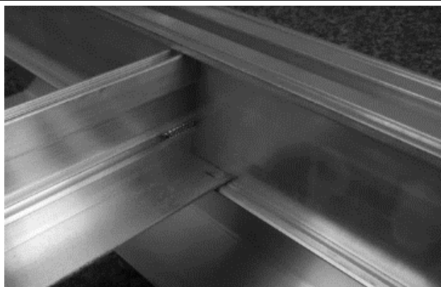
Détail de l'assemblage de l'entretoise
