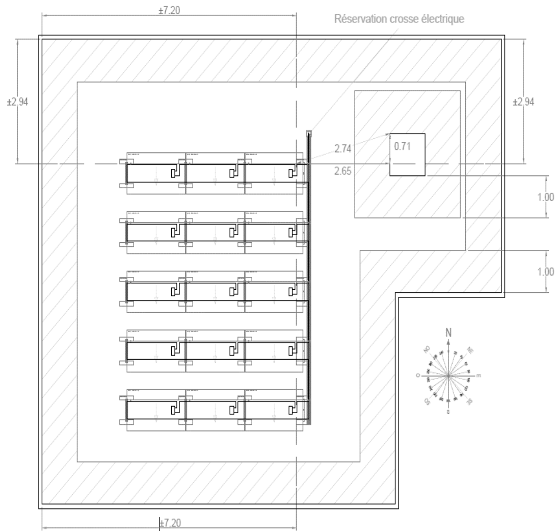
Figure 17 – Exemple de plan Tout Corps d'Etat
