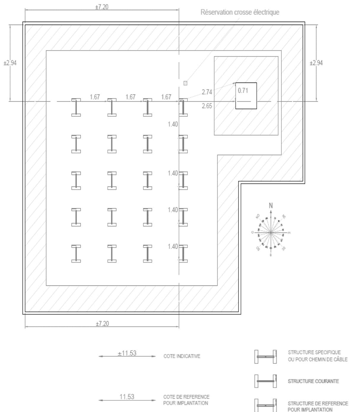
Figure 18 – Exemple de plan d'implantation des ossatures supports iNova PV Lite
