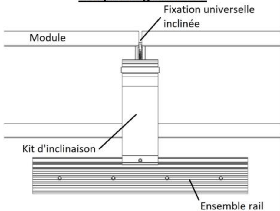
Figure 32 - Assemblage rail / kit d'inclinaison / module
