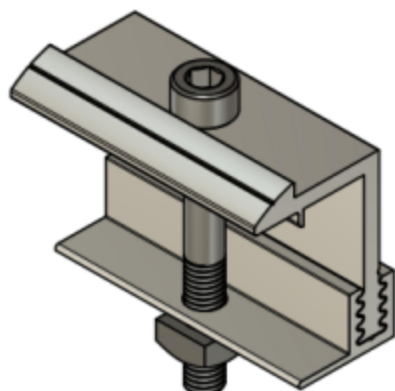
Figure 15 - Fixation Extérieure inclinée du kit d'inclinaison du procédé ROOF-SOLAR BITUME TANDTU – Plat & Incliné600
