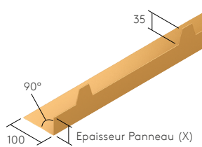
Closoir cranté
