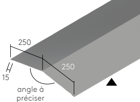
Sous-faîtière
